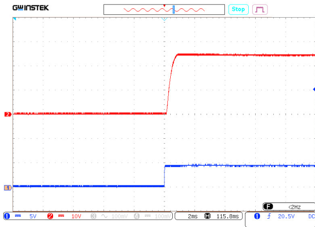
Рис. 26. Осциллограмма установления выходного напряжения с момента подачи команды дистанционного управления. Луч 1 (синий) – напряжение на выводе «ВКЛ». Масштаб 5 В/дел. Луч 2 (красный) – выходное напряжение. Масштаб 10 В/дел. Развертка 2 мс/дел.
