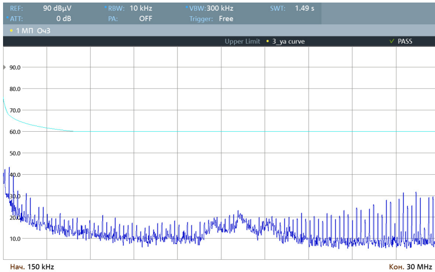
Рис. 36. Диапазон 0,15..30 МГц.
