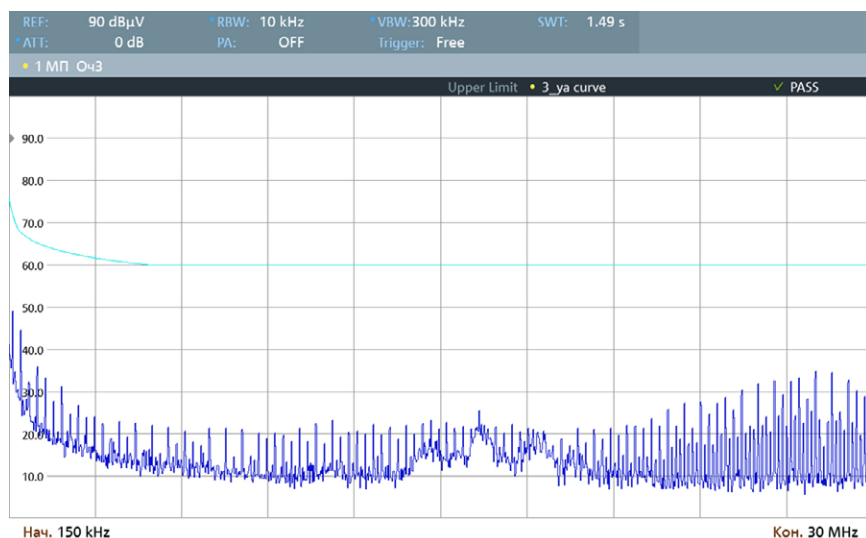
Рис. 34. Диапазон 0,15..30 МГц.
