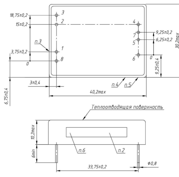
Рис. 42. Модуль двухканальный в корпусе без фланцев.
