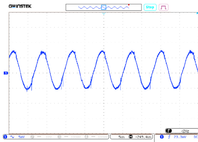
Рис. 28. Осциллограмма пульсаций выходного напряжения.
