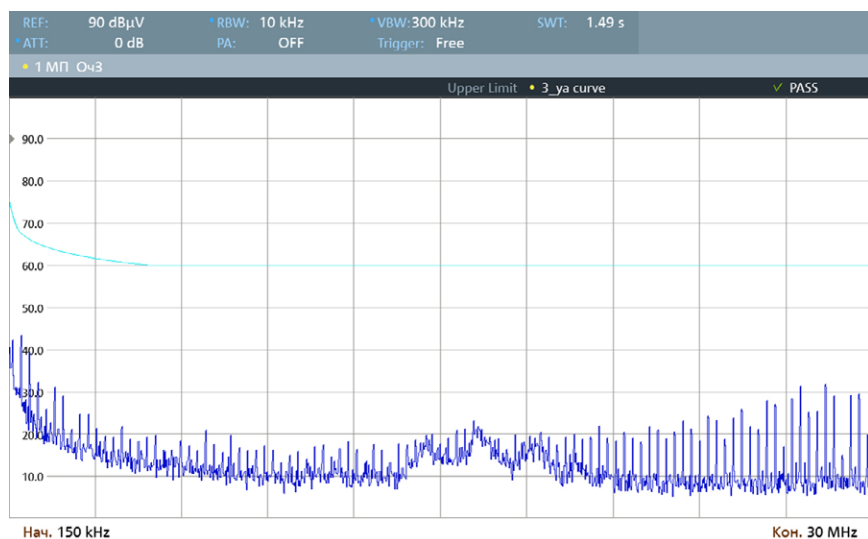
Рис. 36. Диапазон 0,15..30 МГц.
