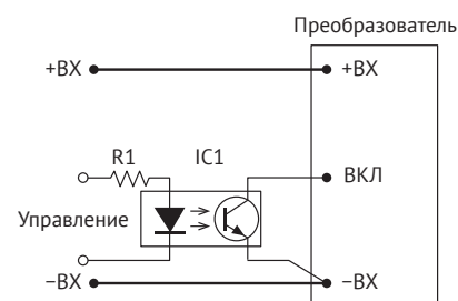
Рис. 9. ВКЛ/ВЫКЛ с помощью оптрона.
