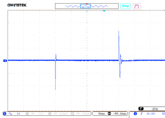
Рис. 29. Осциллограмма переходного отклонения выходного напряжения при изменении выходного тока с 50% до 100 %.
