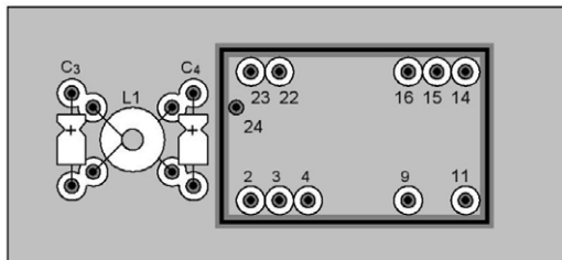
Рис. 5. Вид сверху.
