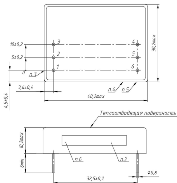
Рис. 40. Модуль одноканальный в корпусе без фланцев. Исполнение II.
