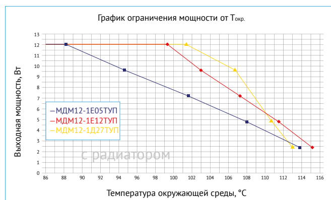
Рис. 21. График ограничения мощности от T_{окр.} с применением радиатора БКЯЮ.752695.033 ( S=74 \text{ см}^2 ).
