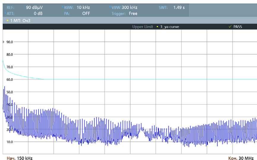
Рис. 35. Диапазон 0,15..30 МГц.
