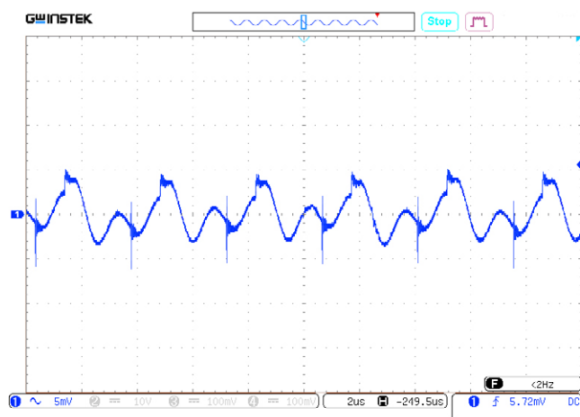
Рис. 32. Осциллограмма пульсаций выходного напряжения.
