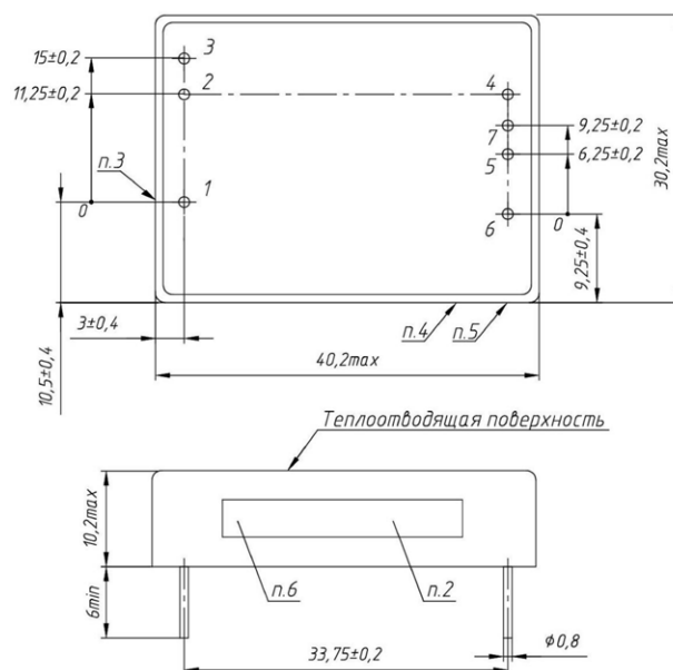
Рис. 44. Модуль двухканальный в корпусе без фланцев. Исполнение II.
