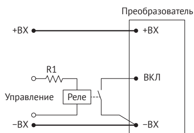
Рис. 7. ВКЛ/ВЫКЛ с помощью реле.
