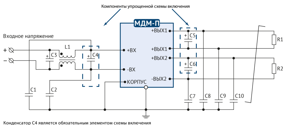
Рис. 3. Типовая схема подключения двухканального модуля.
