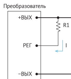
Рис. 11. Снижение U_{\text{вых}} .
