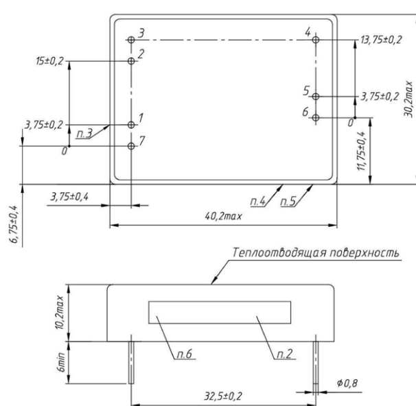
Рис. 38. Модуль одноканальный в корпусе без фланцев.
