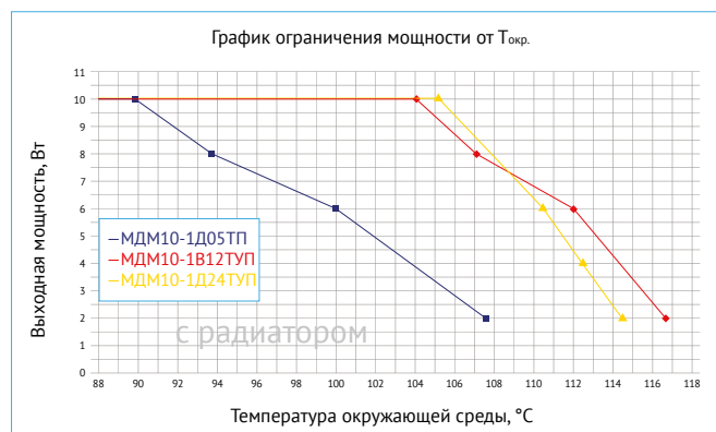
Рис. 19. График ограничения мощности от T_{окр.} с применением радиатора БКЯЮ.752695.033 ( S=74 \text{ см}^2 ).
