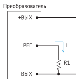
Рис. 10. Увеличение U_{\text{вых}} .
