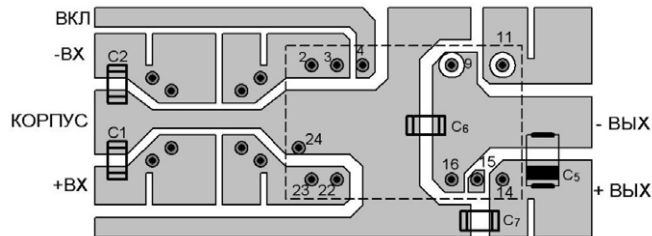
Рис. 6. Вид снизу.
