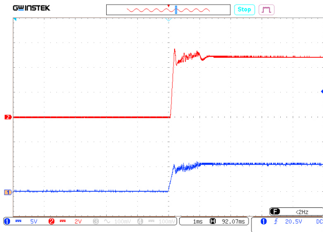
Рис. 30. Осциллограмма установления выходного напряжения с момента подачи команды дистанционного управления. Луч 1 (синий) – напряжение на выводе «VKЛ». Масштаб 5 В/дел. Луч 2 (красный) – выходное напряжение. Масштаб 2 В/дел. Развертка 1 мс/дел.
