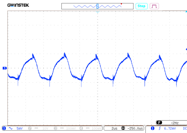
Рис. 24. Осциллограмма пульсаций выходного напряжения. Масштаб 5 мВ/дел. Развертка 2 мкс/дел.
