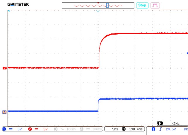
Рис. 22. Осциллограмма установления выходного напряжения с момента подачи команды дистанционного управления. Луч 1 (синий) – напряжение на выводе «ВКЛ». Масштаб 5 В/дел. Луч 2 (красный) – выходное напряжение. Масштаб 5 В/дел. Развертка 5 мс/дел.
