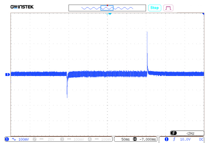
Рис. 25. Осциллограмма переходного отклонения выходного напряжения при изменении выходного тока с 50% до 100%. Масштаб 100 мВ/дел. Развертка 50 мс/дел.
