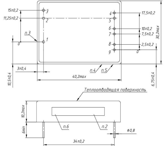
Рис. 48. Модуль трехканальный в корпусе без фланцев. Исполнение II.
