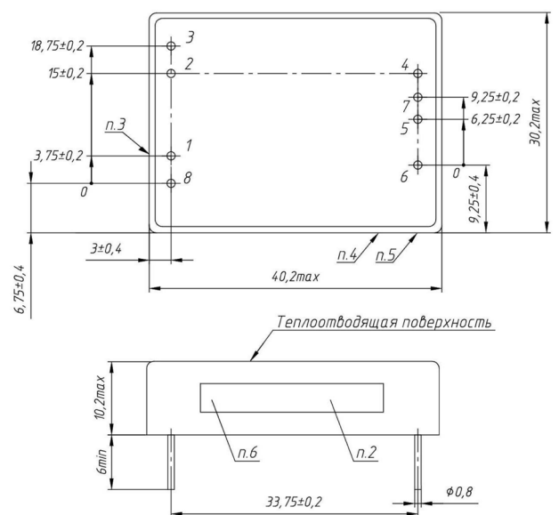
Рис. 42. Модуль двухканальный в корпусе без фланцев.
