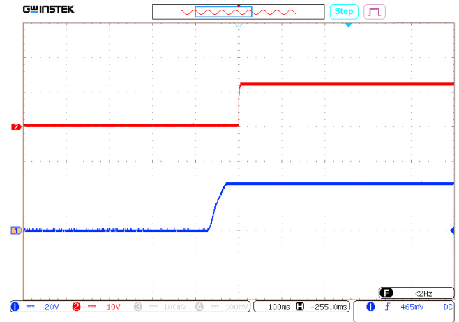
Рис. 23. Осциллограмма установления выходного напряжения с момента подачи входного напряжения. Луч 1 (синий) – входное напряжение. Масштаб 20 В/дел. Луч 2 (красный) – выходное напряжение. Масштаб 10 В/дел. Развертка 100 мс/дел.
