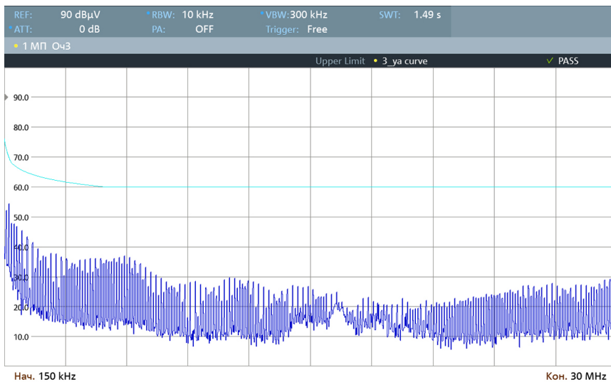
Рис. 35. Диапазон 0,15..30 МГц.
