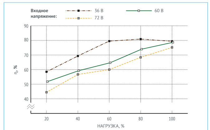
Рис. 16. МДМ6-1Д27МУП.
