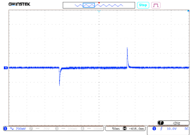
Рис. 24. Осциллограмма переходного отклонения выходного напряжения при изменении выходного тока с 50% до 100%. Масштаб 200 мВ/дел. Развертка 50 нс/дел.
