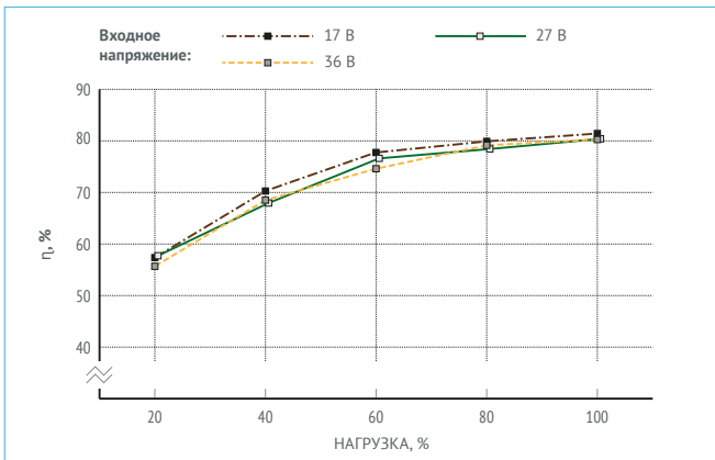
Рис. 13. МДМ6-1В37ТУП.
