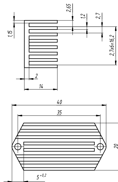
Рис. 39. БКЯЮ.752694.008.
