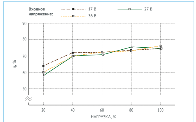
Рис. 12. МДМ6-1В30ТУП.
