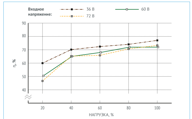
Рис. 14. МДМ6-1Д05МУП.
