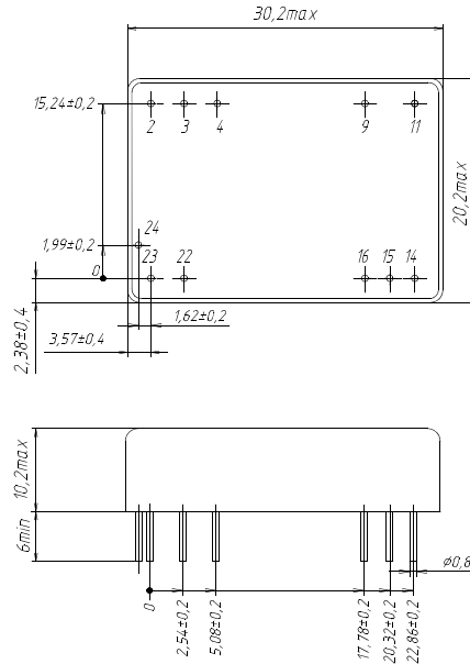
Рис. 35. Модуль одноканальный в корпусе без фланцев.
