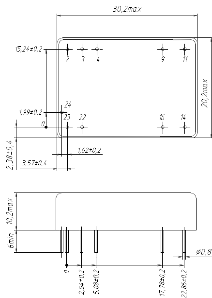
Рис. 37. Модуль двухканальный в корпусе без фланцев.
