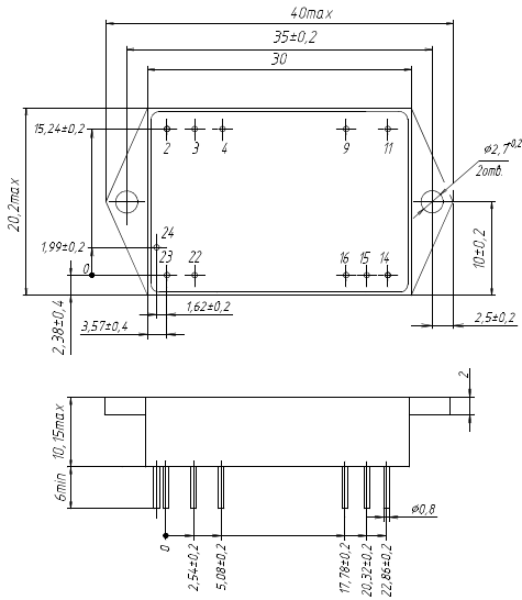
Рис. 34. Модуль одноканальный в корпусе с фланцами (индекс «У»).
