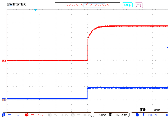
Рис. 29. Осциллограмма установления выходного напряжения с момента подачи команды дистанционного управления. Луч 1 (синий) – напряжение на выводе «VKЛ». Масштаб 5 В/дел. Луч 2 (красный) – выходное напряжение. Масштаб 10 В/дел. Развертка 50 мс/дел.
