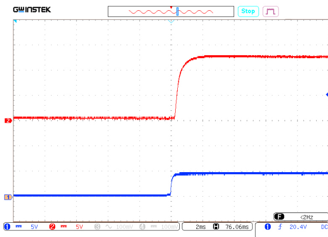
Рис. 20. Осциллограмма установления выходного напряжения с момента подачи команды дистанционного управления. Луч 1 (синий) — напряжение на выходе «ВКЛ». Масштаб 5 В/дел. Луч 2 (красный) — выходное напряжение. Масштаб 5 В/дел. Развертка 2 мс/дел.
