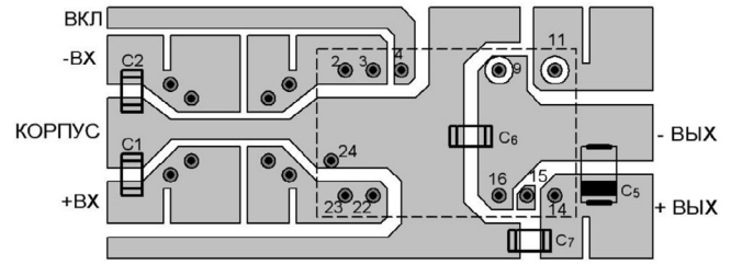
Рис. 5. Вид снизу.
