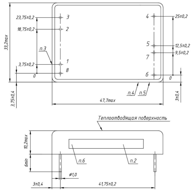
Рис. 39. Модуль двухканальный в корпусе без фланцев.
