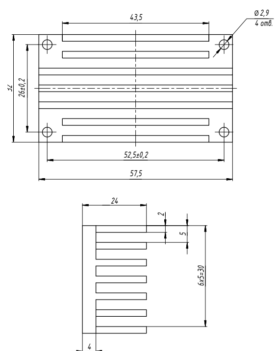
Рис. 45. БКЯЮ.752695.262-01.
