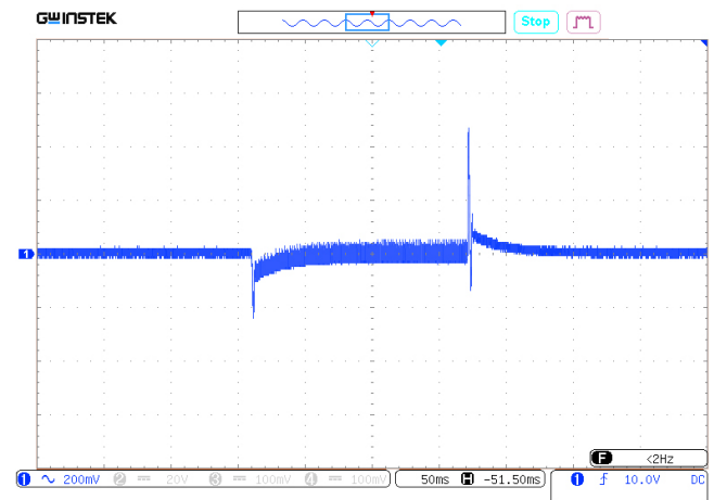
Рис. 30. Осциллограмма переходного отклонения выходного напряжения при изменении выходного тока с 50% до 100%. Масштаб 200 мВ/дел. Развертка 50 мс/дел.
