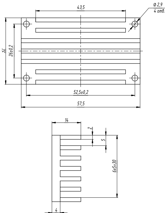
Рис. 43. БКЯЮ.752695.262.
