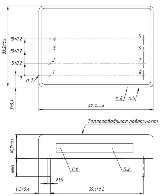
Рис. 41. Модуль двухканальный в корпусе без фланцев. Исполнение II.
