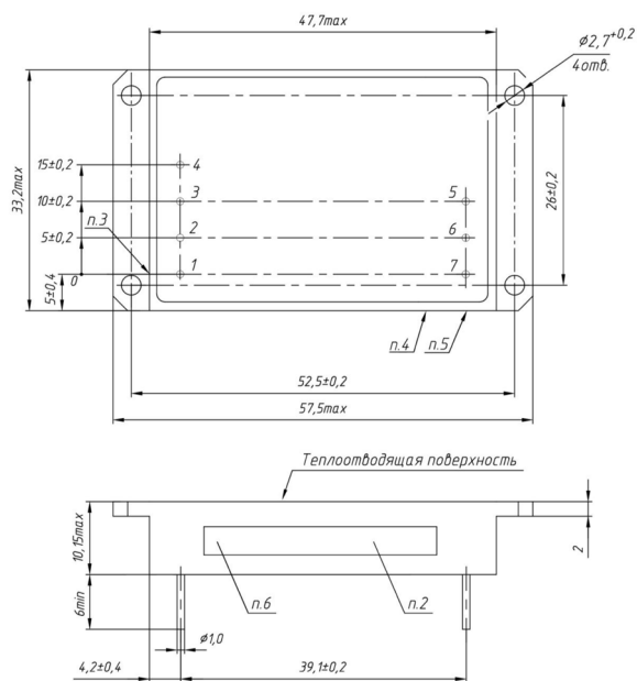
Рис. 36. Модуль одноканальный в корпусе с фланцами (индекс «У»).
