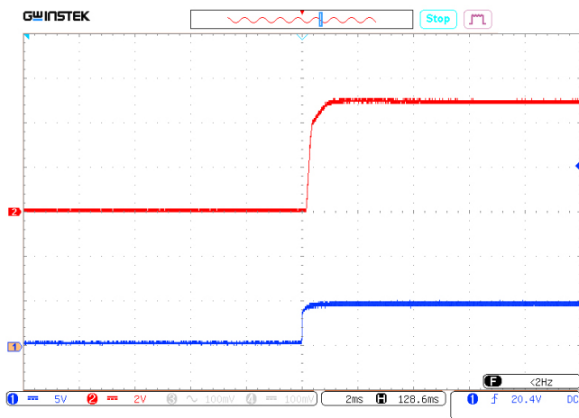
Рис. 27. Осциллограмма установления выходного напряжения с момента подачи команды дистанционного управления. Луч 1 (синий) – напряжение на выводе «ВКЛ». Масштаб 5 В/дел. Луч 2 (красный) – выходное напряжение. Масштаб 2 В/дел. Развертка 2 мс/дел.
