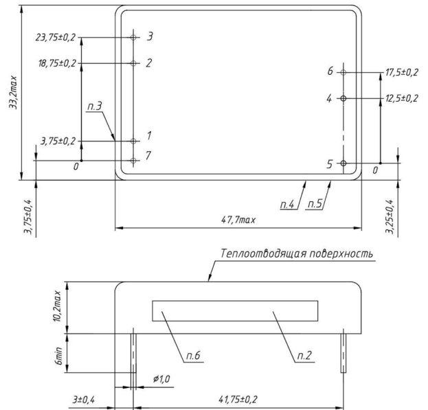
Рис. 35. Модуль одноканальный в корпусе без фланцев.
