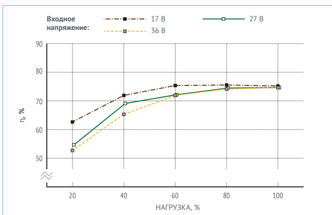
Рис. 11. МДМ20-1В05ТУП.
