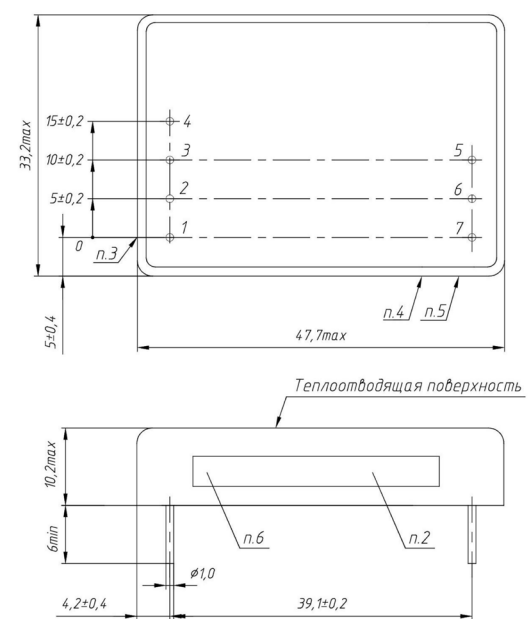
Рис. 37. Модуль одноканальный в корпусе без фланцев.
