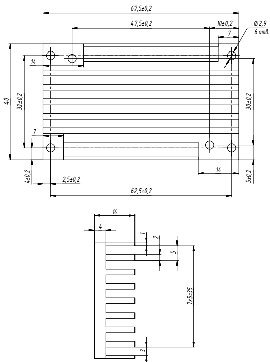
Рис. 36. БКЯЮ.752695.263.
