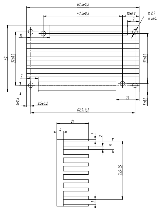
Рис. 38. БКЯЮ.752695.263-01.
