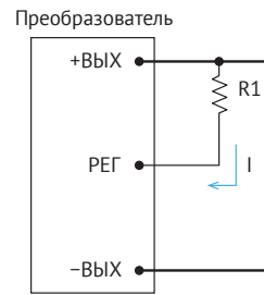
Рис. 10. Снижение I_{\text{вых}} .
