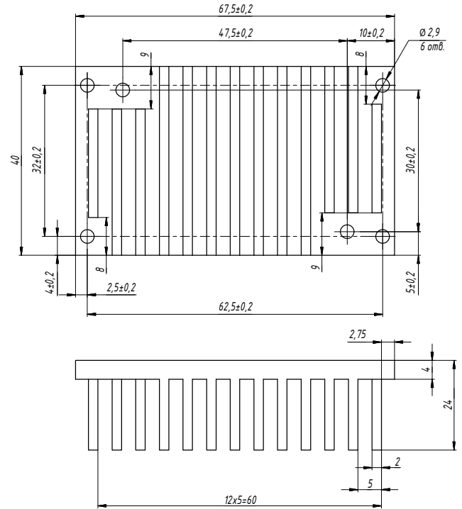
Рис. 37. БКЯЮ.752695.055-01.
