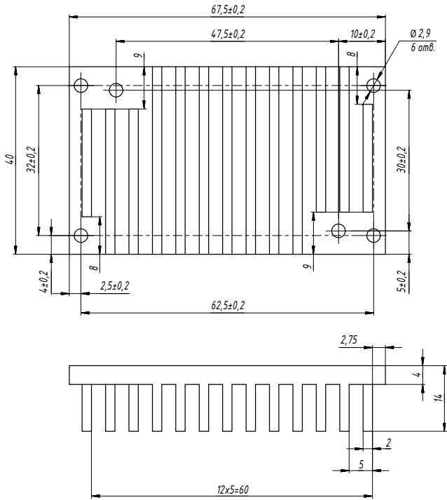
Рис. 35. БКЯЮ.752695.055.
