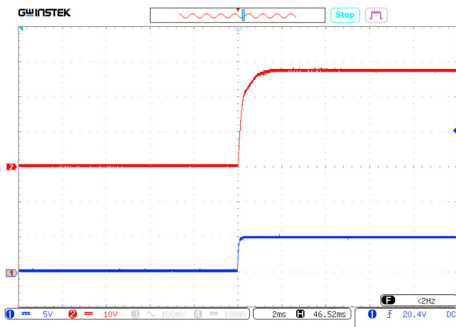
Рис. 23. Осциллограмма установления выходного напряжения с момента подачи команды дистанционного управления. Луч 1 (синий) – напряжение на выводе «VKЛ». Масштаб 5 В/дел. Луч 2 (красный) – выходное напряжение. Масштаб 10 В/дел. Развертка 2 мс/дел.
