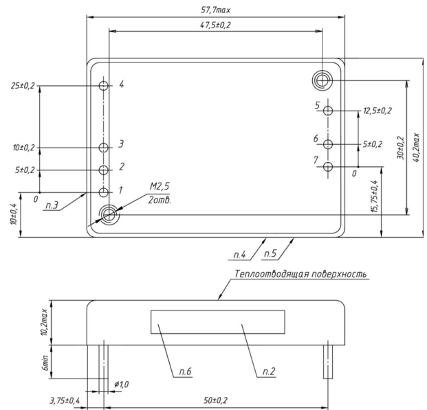
Рис. 32. Модуль одноканальный в корпусе без фланцев. Исполнение II.
