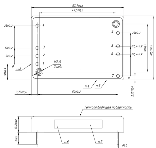
Рис. 34. Модуль двухканальный в корпусе без фланцев.
