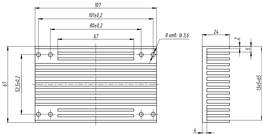
Рис. 31. БКАЮ.752695.265-01.
