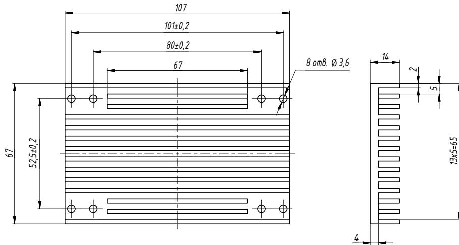
Рис. 30. БКАЮ.752695.265.
