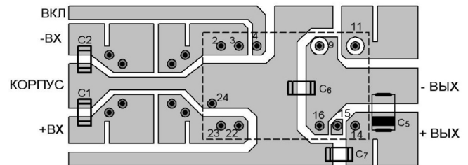
Рис. 4. Вид снизу.
