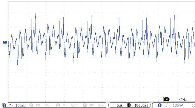
Рис. 19. Осциллограмма пульсаций выходного напряжения. Масштаб 100 мВ/дел. Развертка 1 мкс/дел.
