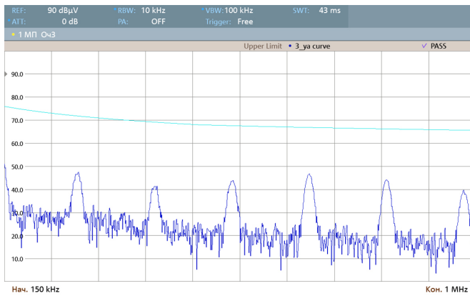
Рис. 29. Диапазон 0,15..1 МГц.
