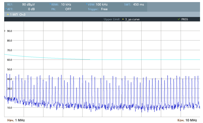
Рис. 30. Диапазон 1..10 МГц.
