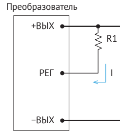
Рис. 7. Снижение U_{\text{ВЫХ}} .
