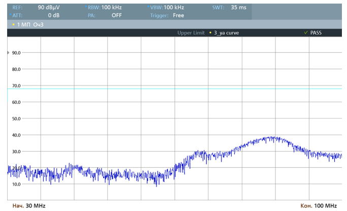
Рис. 28. Диапазон 30..100 МГц.
