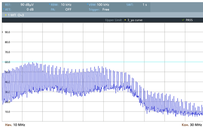
Рис. 27. Диапазон 10..30 МГц.
