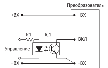
Рис. 5. ВКЛ/ВЫКЛ с помощью оптрона.
