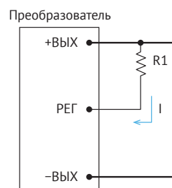
Рис. 7. Снижение U_{ВЫХ} .
