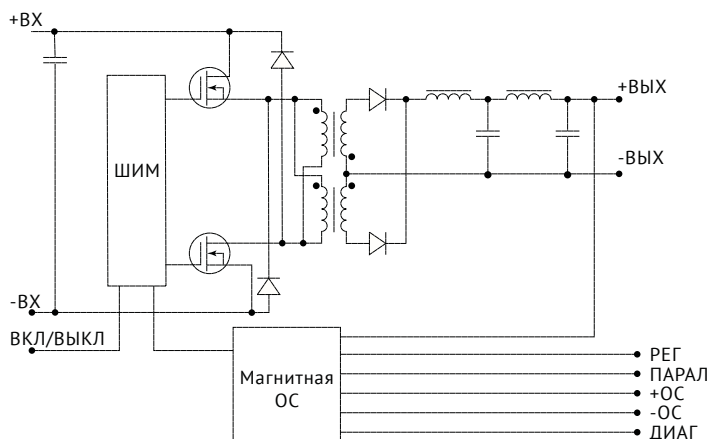
Рис. 1. Функциональная схема МДМ1000-П.
