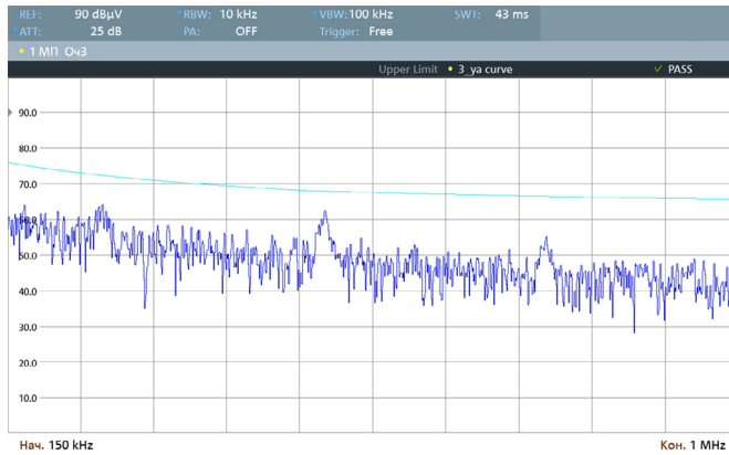
Рис. 17. Диапазон 0,15..1 МГц.
