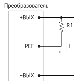
Рис. 7. Снижение U_{ВЫХ} .
