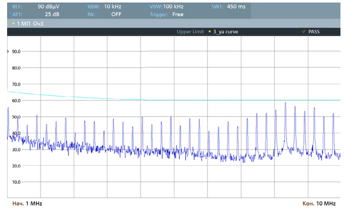
Рис. 18. Диапазон 1..10 МГц.
