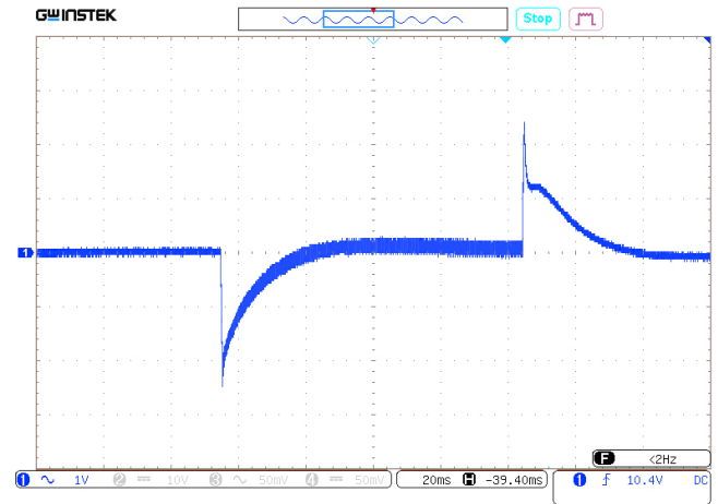
Рис. 16. Осциллограмма переходного отклонения выходного напряжения при изменении выходного тока с 10% до 100 %.
