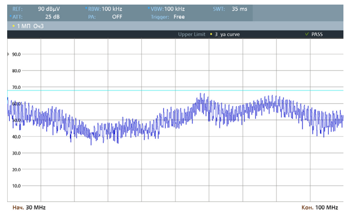
Рис. 20. Диапазон 30..100 МГц.
