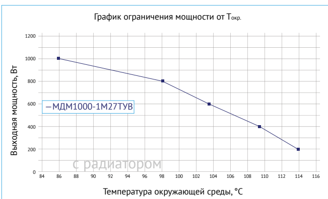
Рис. 12. График ограничения мощности от T_{окр} с применением радиатора БКЯЮ.752695.067 ( S=1890 \text{ см}^2 ) с принудительным обдувом, скорость воздушного потока 3,5 м/с.
