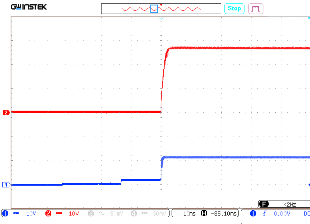
Рис. 13. Осциллограмма установления выходного напряжения с момента подачи команды дистанционного управления.
