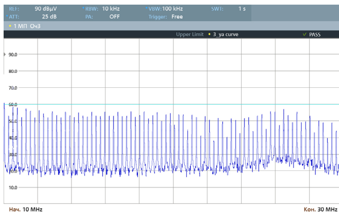
Рис. 19. Диапазон 10..30 МГц.
