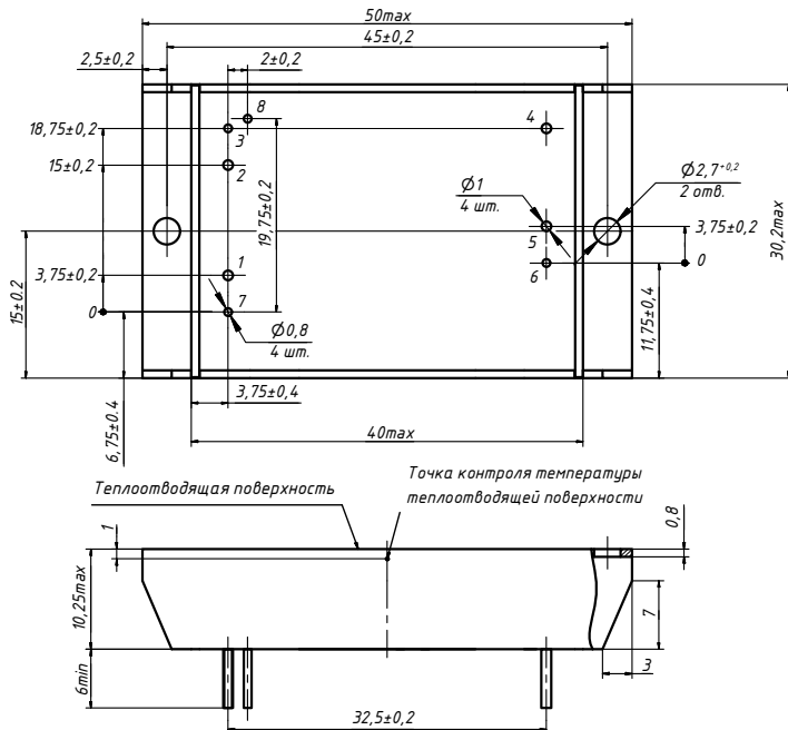
Рис. 42. Исполнение в усиленном корпусе с фланцами для МДМ40-Р, МДМ50-Р.
