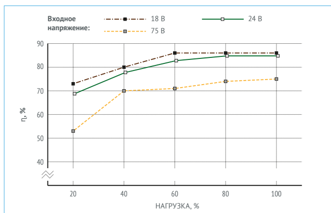
Рис. 21. МДМ50-1Ш09ТУР.
