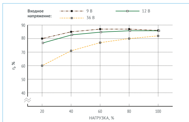
Рис. 12. МДМ50-1Б3,3ТУР.
