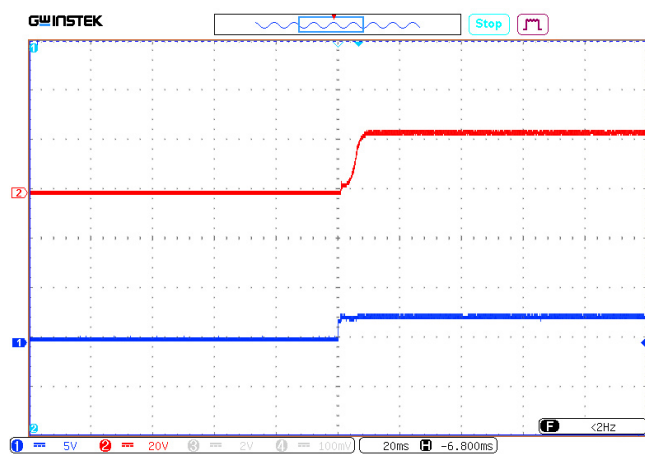
Рис. 34. Осциллограмма установления выходного напряжения с момента подачи команды дистанционного управления. Луч 1 (синий) — напряжение на выводе «ВКЛ». Масштаб 5 В/дел. Луч 2 (красный) — выходное напряжение. Масштаб 20 В/дел. Развертка 20 мс/дел.
