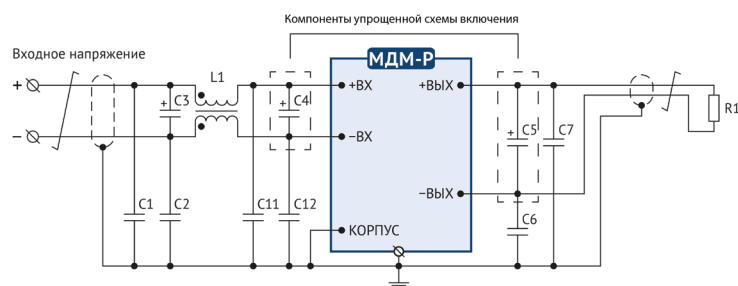
Рис. 2. Типовая схема подключения.
