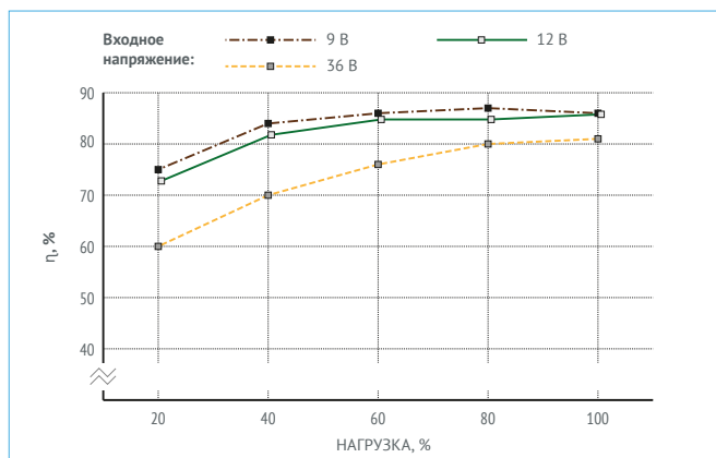
Рис. 18. МДМ50-1527ТУР.
