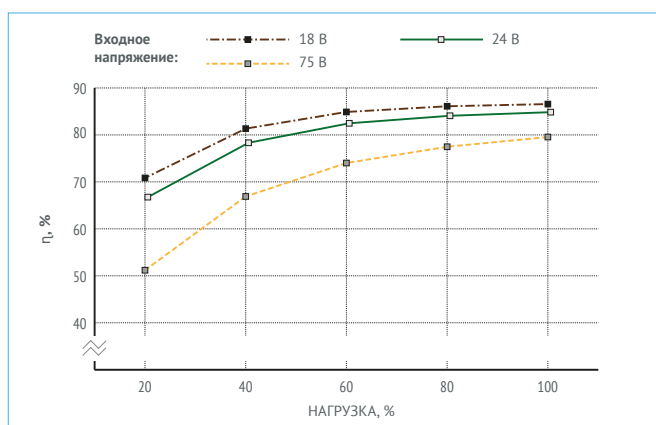
Рис. 19. МДМ50-1Ш3,3ТУР.
