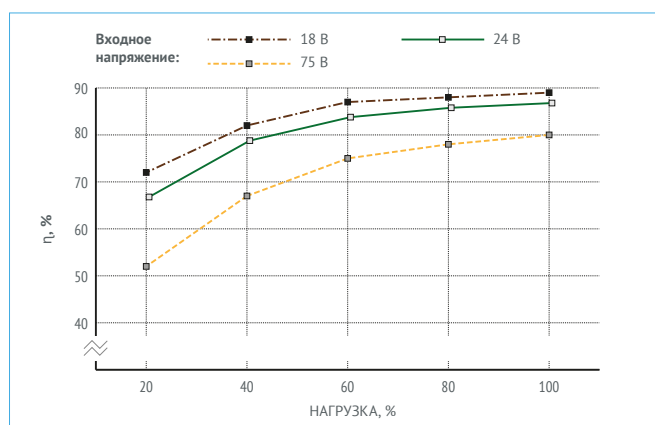
Рис. 20. МДМ50-1Ш05ТУР.
