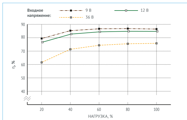
Рис. 14. МДМ50-1Б09ТУР.
