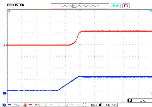
Рис. 35. Осциллограмма установления выходного напряжения с момента подачи входного напряжения. Луч 1 (синий) — входное напряжение. Масштаб 20 В/дел. Луч 2 (красный) — выходное напряжение. Масштаб 20 В/дел. Развертка 10 мс/дел.
