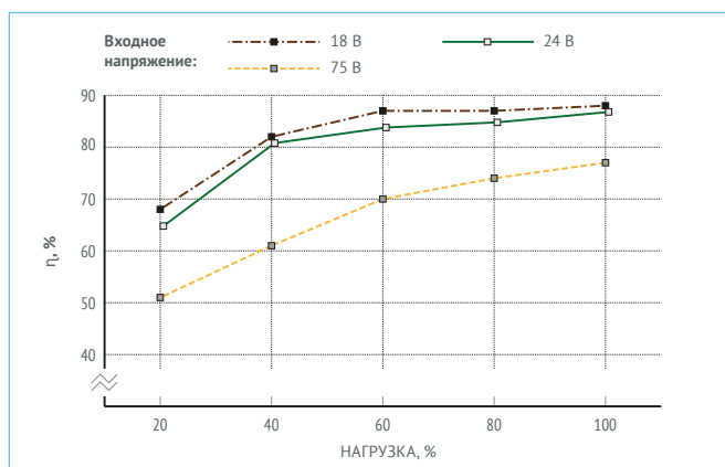
Рис. 23. МДМ50-1Ш15ТУР.
