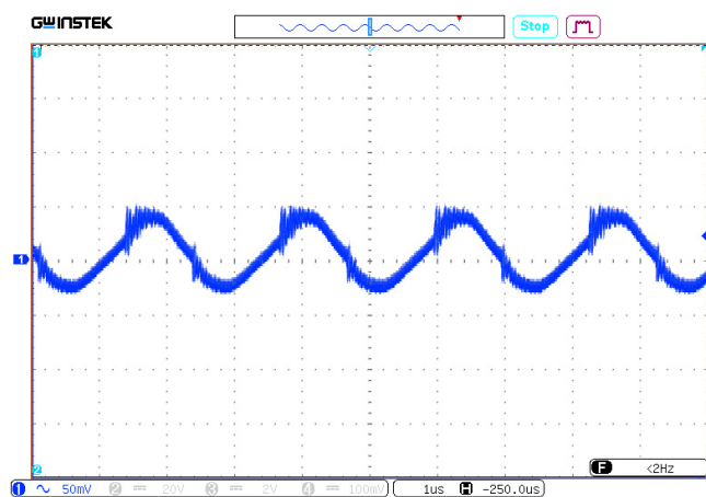
Рис. 36. Осциллограмма пульсаций выходного напряжения. Масштаб 50 мВ/дел. Развертка 1 мс/дел.
