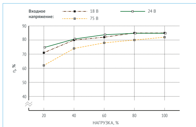
Рис. 24. МДМ50-1Ш24ТУР.
