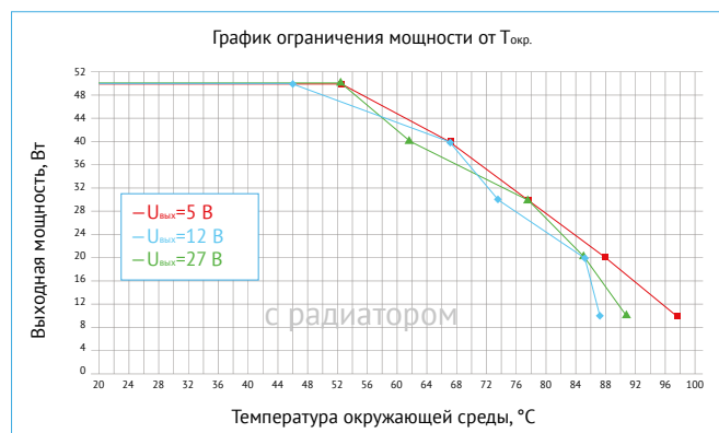
Рис. 27. График ограничения мощности от T_{ОКР.} с применением радиатора БКЯЮ.752695.033 ( S=74 \text{ см}^2 ).
