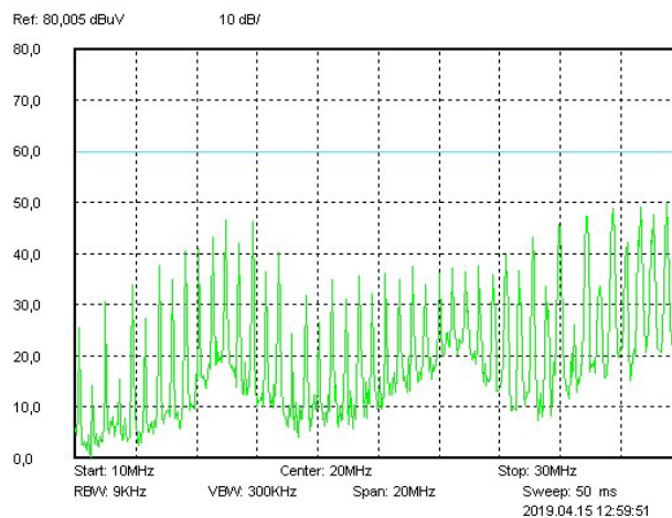
Рис. 39. Диапазон 10..30 МГц.
