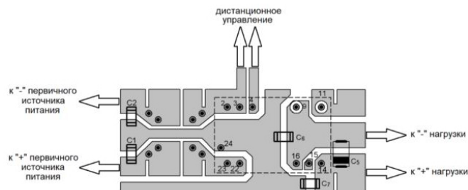
Рис. 4. Вид снизу.
