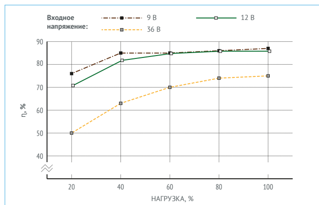
Рис. 15. МДМ50-1Б12ТУР.
