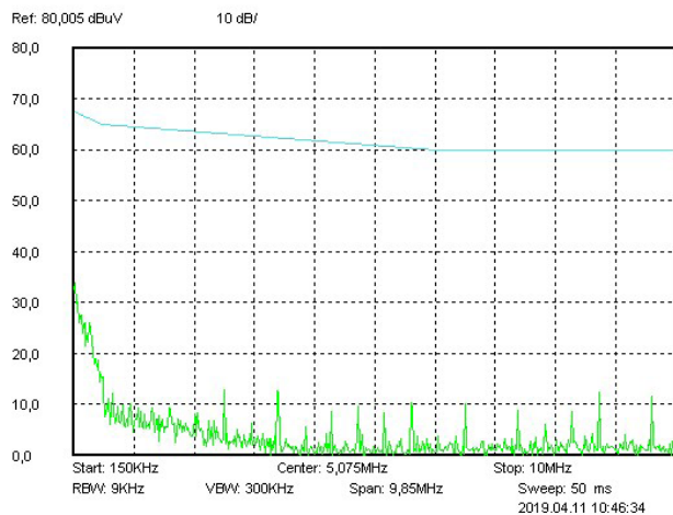
Рис. 40. Диапазон 0,15..10 МГц.
