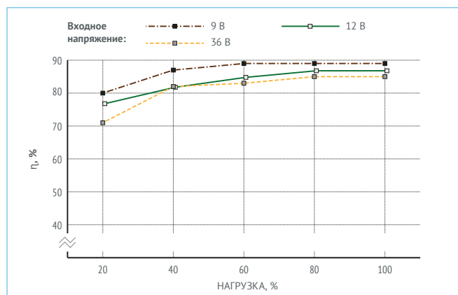
Рис. 17. МДМ50-1Б24ТУР.
