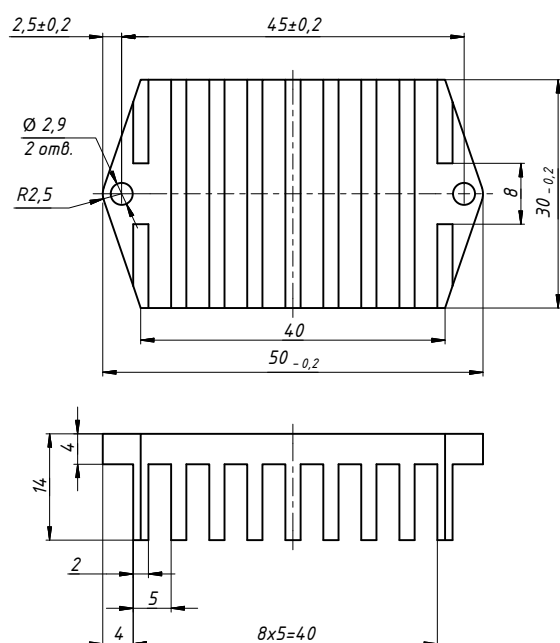
Рис. 43. БКЯЮ.752695.033.
