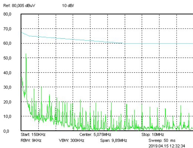
Рис. 38. Диапазон 0,15..10 МГц.
