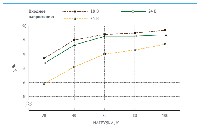
Рис. 22. МДМ50-1Ш12ТУР.
