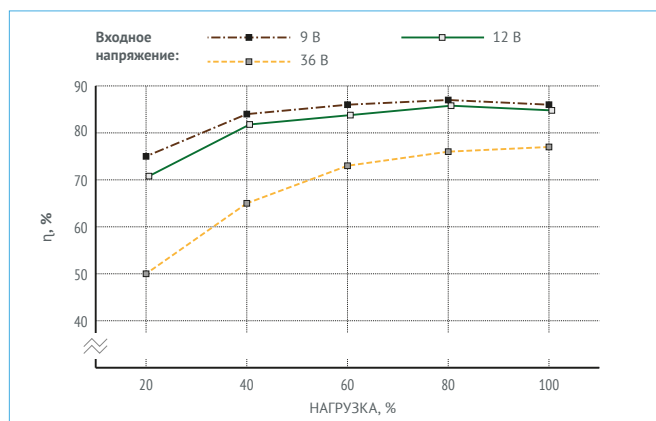
Рис. 16. МДМ50-1Б15ТУР.
