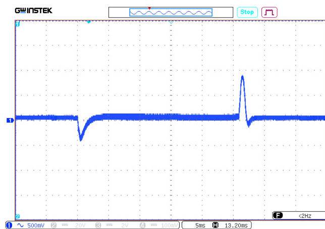
Рис. 37. Осциллограмма переходного отклонения выходного напряжения при изменении выходного тока с 50% до 100 %. Масштаб 500 В/дел. Развертка 5 мс/дел.
