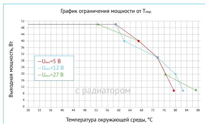
Рис. 29. График ограничения мощности от T_{ОКР.} с применением радиатора БКЯЮ.752695.033 ( S=74 \text{ см}^2 ).
