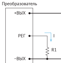
Рис. 9. Увеличение U_{\text{вых}} .
