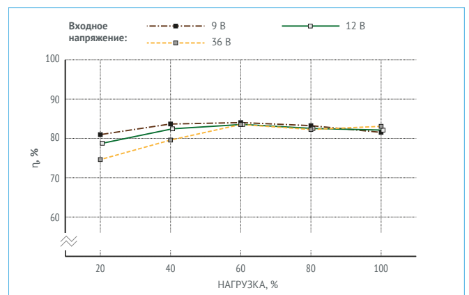
Рис. 26. МДМ25-1Б09ТУР.
