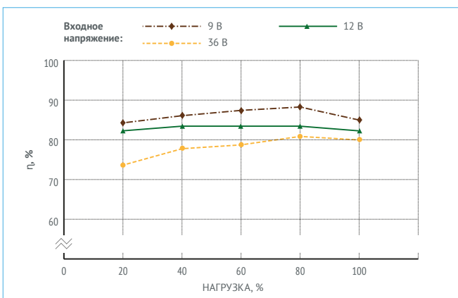
Рис. 25. МДМ25-1Б05ТУР.
