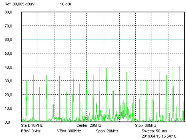
Рис. 49. Диапазон 10..30 МГц.
