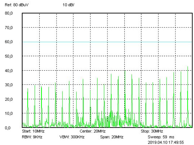
Рис. 51. Диапазон 10..30 МГц.
