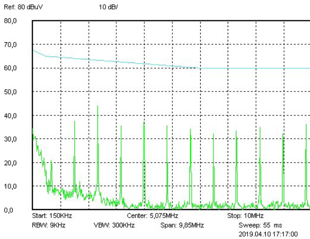
Рис. 48. Диапазон 0,15..10 МГц.
