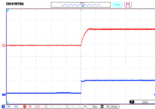
Рис. 44. Осциллограмма установления выходного напряжения с момента подачи команды дистанционного управления. Луч 1 (синий) — напряжение на выводе «VKЛ». Масштаб 5 В/дел. Луч 2 (красный) — выходное напряжение. Масштаб 20 В/дел. Развертка 5 мс/дел.
