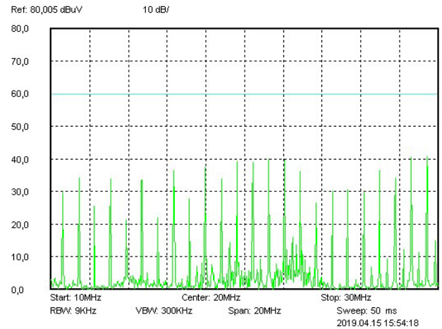
Рис. 49. Диапазон 10..30 МГц.
