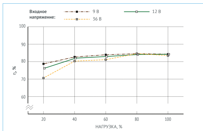
Рис. 27. МДМ25-1Б15ТУР.
