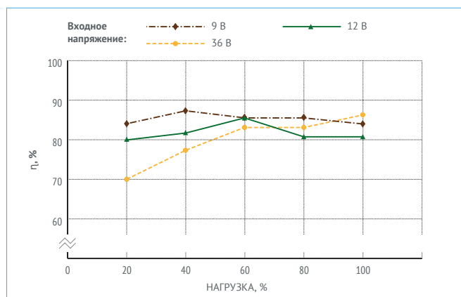
Рис. 28. МДМ25-1Б24ТУР.
