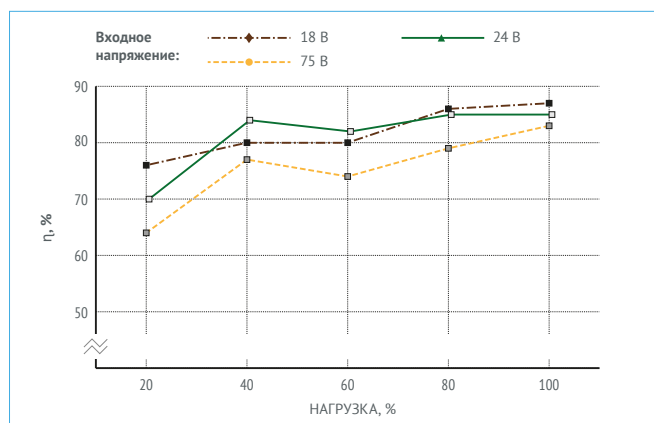
Рис. 23. МДМ15-1Ш24ТУР.
