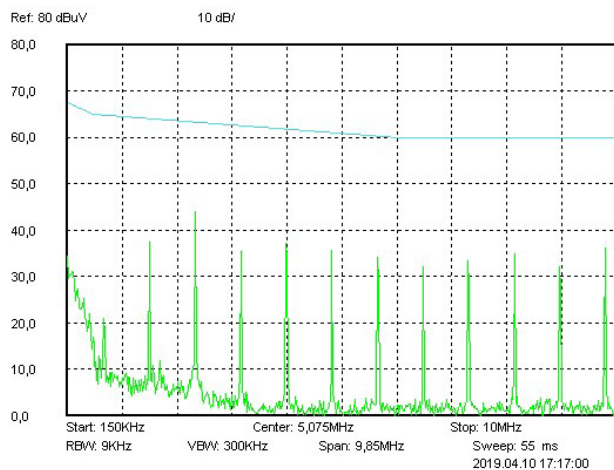
Рис. 48. Диапазон 0,15..10 МГц.
