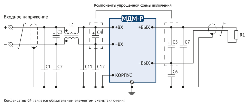
Рис. 3. Типовая схема подключения.
