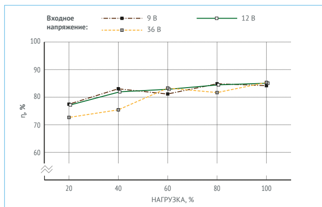
Рис. 29. МДМ25-1Б27ТУР.
