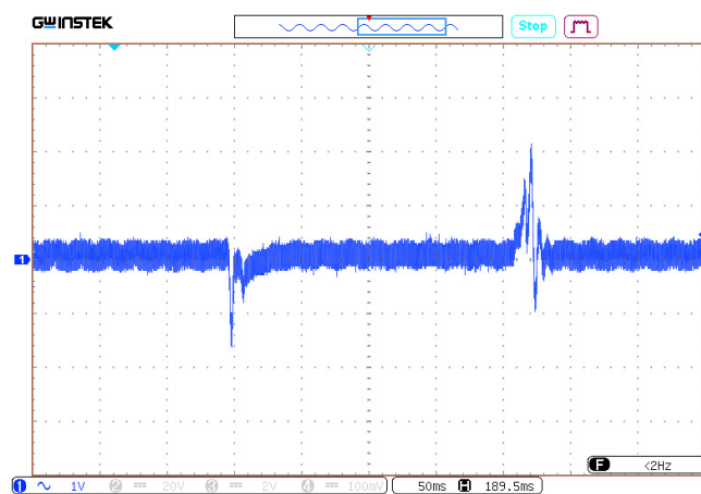
Рис. 47. Осциллограмма переходного отклонения выходного напряжения при изменении выходного тока с 50% до 100 %.
