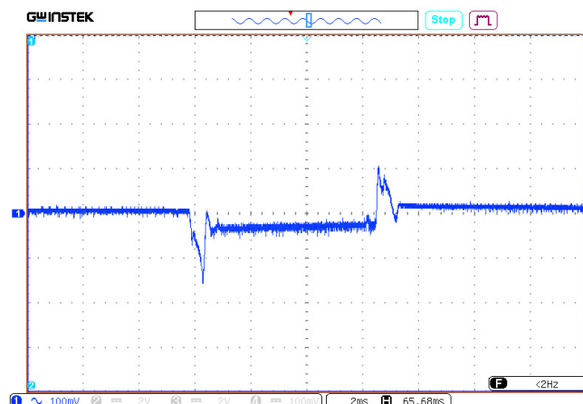
Рис. 43. Осциллограмма переходного отклонения выходного напряжения при изменении выходного тока с 50% до 100 %.
