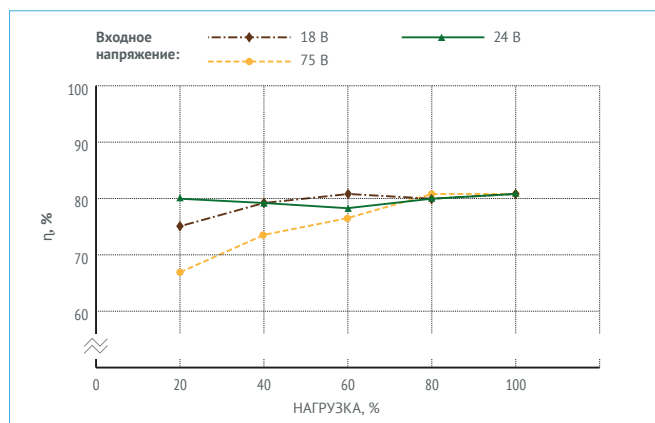
Рис. 31. МДМ25-1Ш05ТУР.
