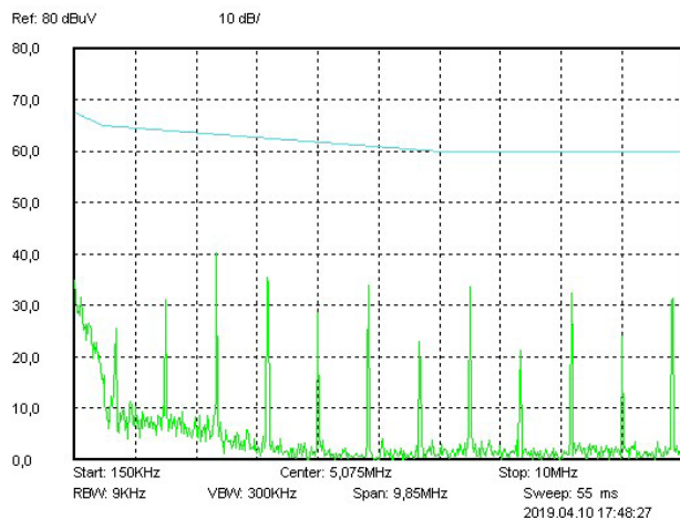
Рис. 50. Диапазон 0,15..10 МГц.
