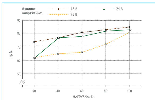
Рис. 22. МДМ15-1Ш15ТУР.
