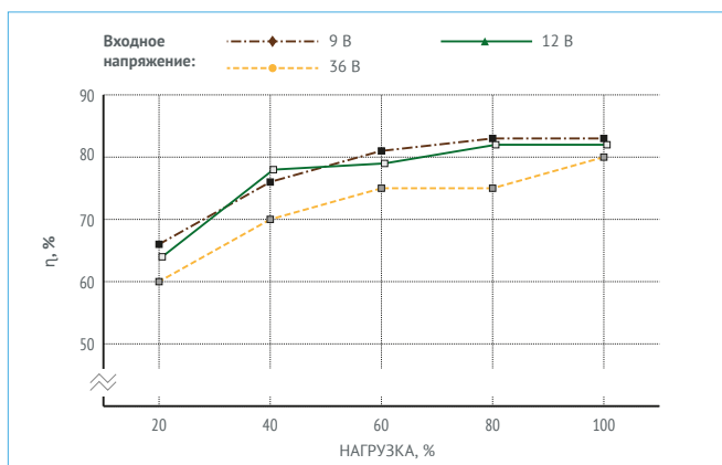
Рис. 15. МДМ15-1Б15ТУР.
