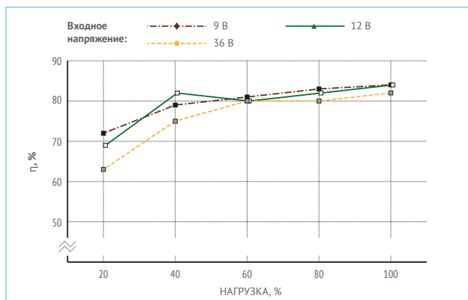
Рис. 17. МДМ15-1627ТУР.
