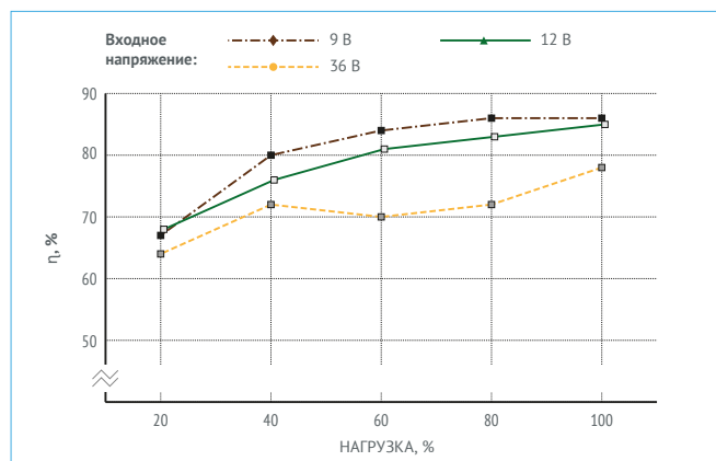
Рис. 14. МДМ15-1Б12ТУР.
