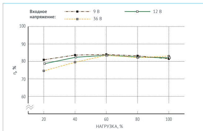
Рис. 26. МДМ25-1Б09ТУР.
