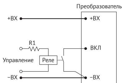
Рис. 6. ВКЛ/ВЫКЛ с помощью реле.
