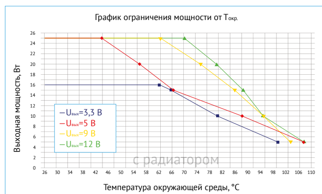
Рис. 39. График ограничения мощности от T_{окр.} с применением радиатора БКЯЮ.752694.008 ( S=74 \text{ см}^2 ).
