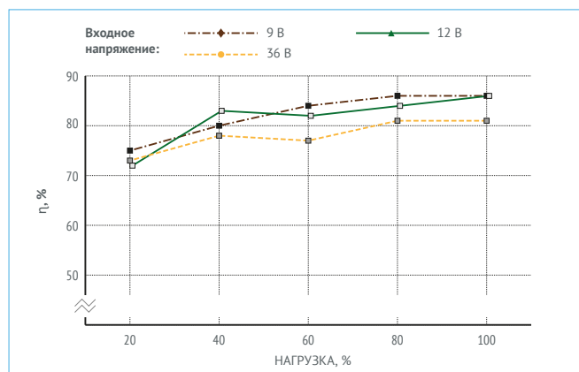
Рис. 16. МДМ15-1Б24ТУР.
