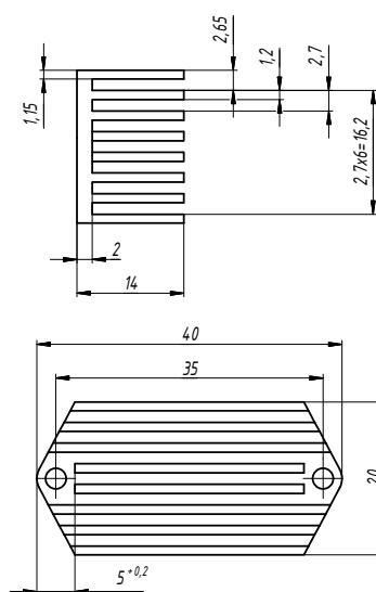
Рис. 54. БКЯЮ.752694.008.
