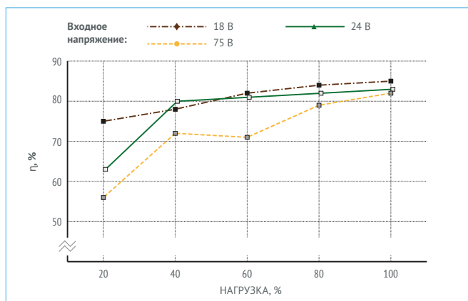
Рис. 24. МДМ15-1Ш27ТУР.
