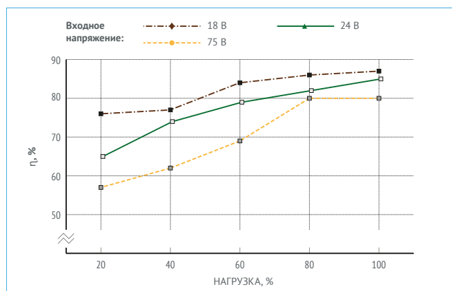
Рис. 21. МДМ15-1Ш12ТУР.
