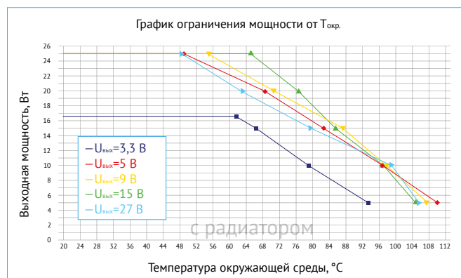
Рис. 37. График ограничения мощности от T_{окр.} с применением радиатора БКЯЮ.752694.008 ( S=74 \text{ см}^2 ).
