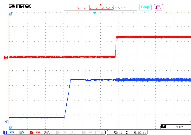
Рис. 45. Осциллограмма установления выходного напряжения с момента подачи входного напряжения.
