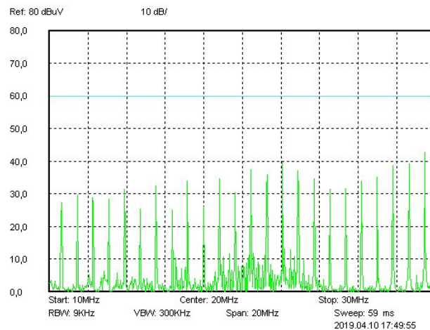
Рис. 51. Диапазон 10..30 МГц.
