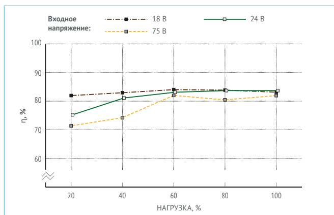
Рис. 32. МДМ25-1Ш09ТУР.
