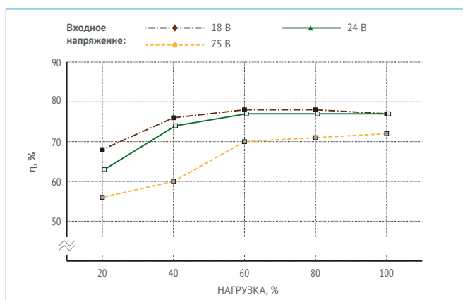
Рис. 18. МДМ15-1Ш3,3ТУР.
