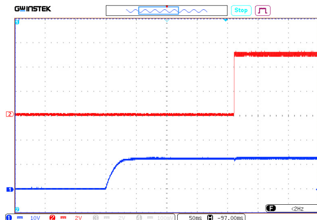
Рис. 41. Осциллограмма установления выходного напряжения с момента подачи входного напряжения.
