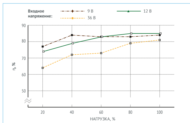
Рис. 12. МДМ15-1Б05ТУР.
