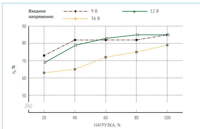
Рис. 13. МДМ15-1Б09ТУР.
