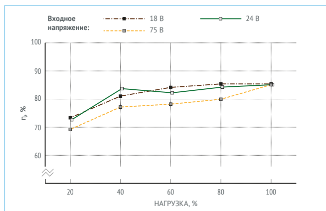
Рис. 35. МДМ25-1Ш27ТУР.
