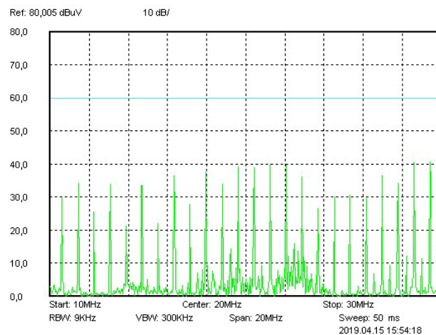
Рис. 49. Диапазон 10..30 МГц.
