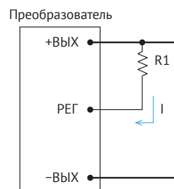
Рис. 10. Снижение U_{\text{вых}} .
