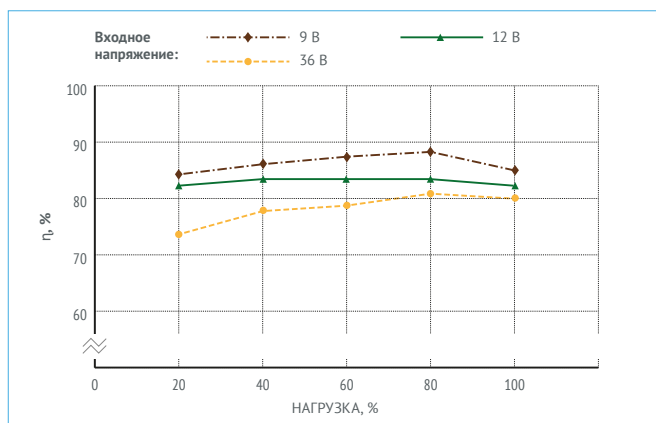
Рис. 25. МДМ25-1Б05ТУР.
