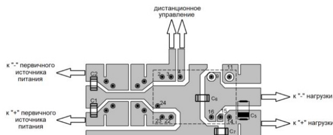
Рис. 5. Вид снизу.
