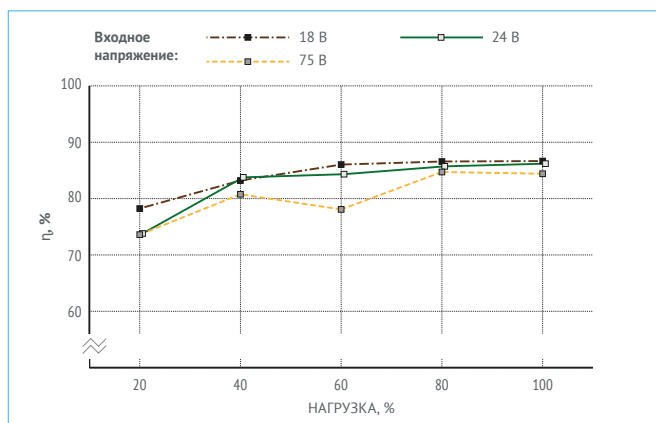
Рис. 34. МДМ25-1Ш24ТУР.
