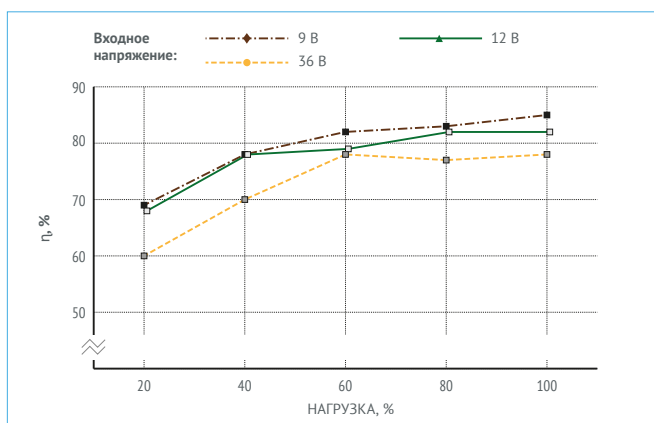
Рис. 11. МДМ15-1Б3,3ТУР.
