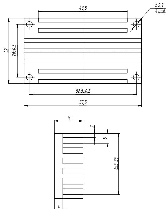
Рис. 40. БКЯЮ.752695.262.
