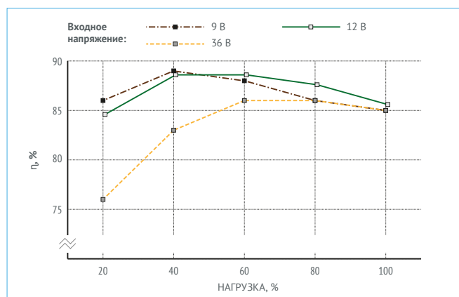
Рис. 13. МДМ100-1Б05СУР.
