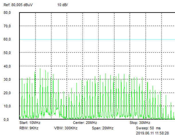
Рис. 37. Диапазон 10..30 МГц.
