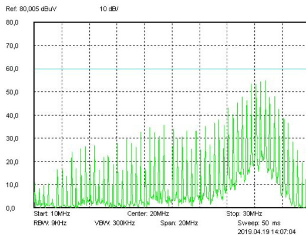
Рис. 35. Диапазон 10..30 МГц.
