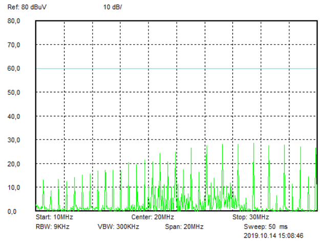
Рис. 64. Диапазон 10..30 МГц.
