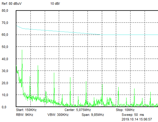
Рис. 63. Диапазон 0,15..10 МГц.
