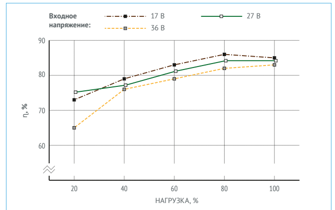
Рис. 33. МДМ10-1В24СР.
