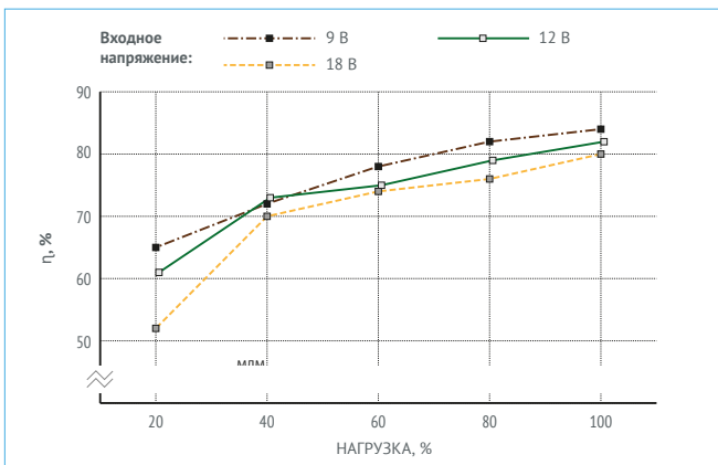
Рис. 14. МДМ6-1А27ТР.
