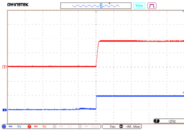
Рис. 55. Осциллограмма установления выходного напряжения с момента подачи команды дистанционного управления.
