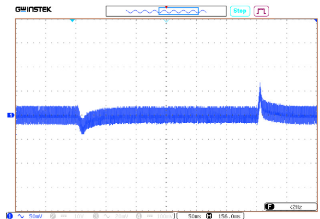
Рис. 46. Осциллограмма переходного отклонения выходного напряжения при изменении выходного тока с 50% до 100%.
