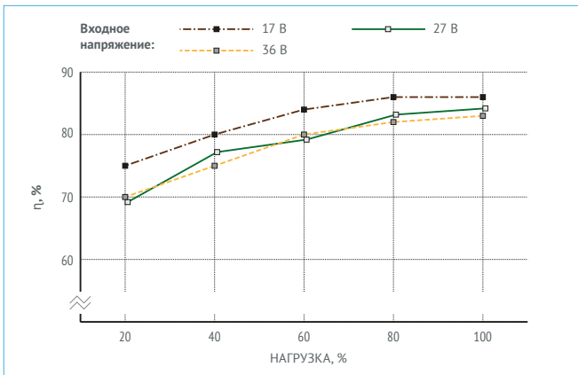
Рис. 31. МДМ10-1В12СР.
