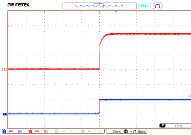
Рис. 51. Осциллограмма установления выходного напряжения с момента подачи команды дистанционного управления. Луч 1 (синий) – напряжение на выводе «VKЛ». Масштаб 5 В/дел. Луч 2 (красный) – выходное напряжение. Масштаб 5 В/дел. Развертка 20 мс/дел.
