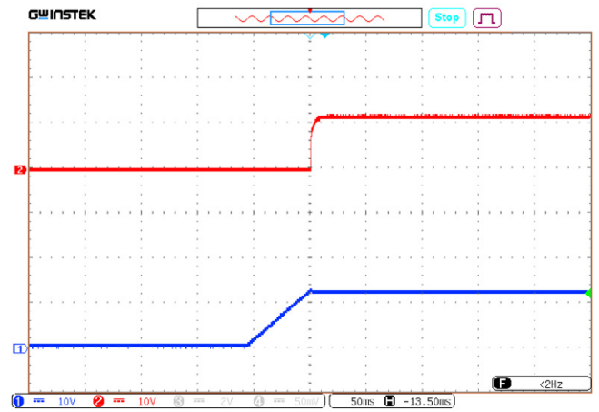
Рис. 52. Осциллограмма установления выходного напряжения с момента подачи входного напряжения. Луч 1 (синий) – входное напряжение. Масштаб 10 В/дел. Луч 2 (красный) – выходное напряжение. Масштаб 10 В/дел. Развертка 50 мс/дел.
