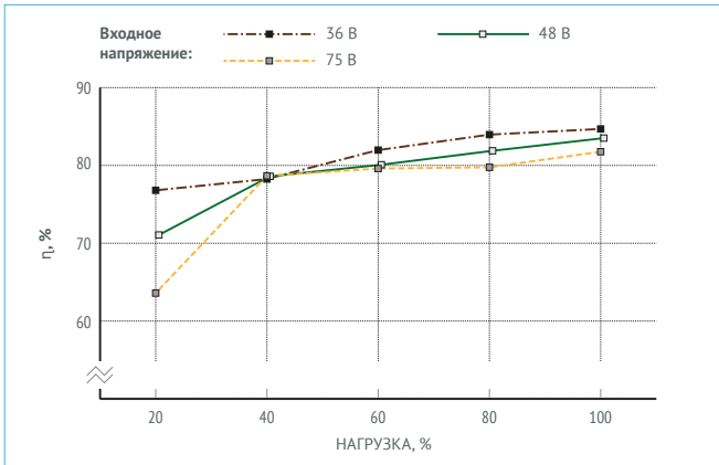
Рис. 36. МДМ10-1Д12СР.
