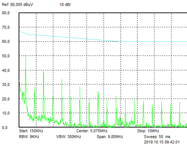
Рис. 69. Диапазон 0,15..10 МГц.
