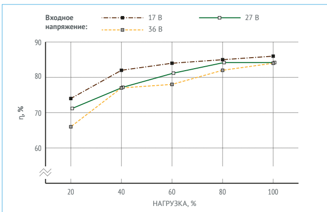
Рис. 32. МДМ10-1В15СР.
