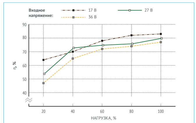
Рис. 20. МДМ6-1В24ТР.
