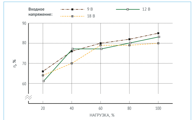
Рис. 13. МДМ6-1А24ТР.
