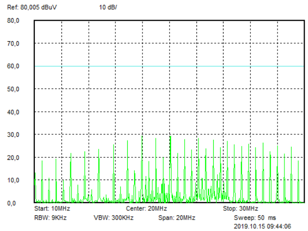
Рис. 70. Диапазон 10..30 МГц.
