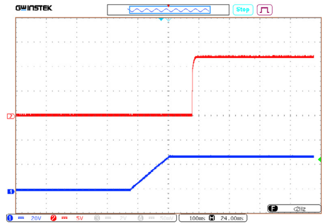
Рис. 48. Осциллограмма установления выходного напряжения с момента подачи входного напряжения. Луч 1 (синий) — входное напряжение. Масштаб 20 В/дел. Луч 2 (красный) — выходное напряжение. Масштаб 5 В/дел. Развертка 100 мс/дел.
