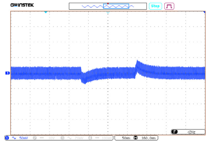
Рис. 58. Осциллограмма переходного отклонения выходного напряжения при изменении выходного тока с 50% до 100%.
