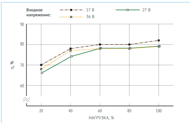
Рис. 29. МДМ10-1В05СР.
