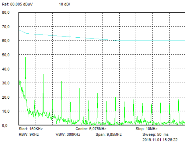
Рис. 67. Диапазон 0,15..10 МГц.
