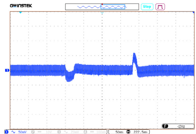
Рис. 62. Осциллограмма переходного отклонения выходного напряжения при изменении выходного тока с 50% до 100%.
