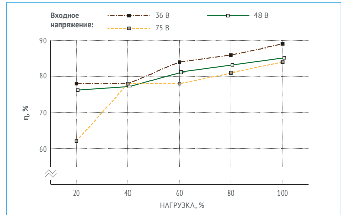
Рис. 37. МДМ10-1Д15СР.
