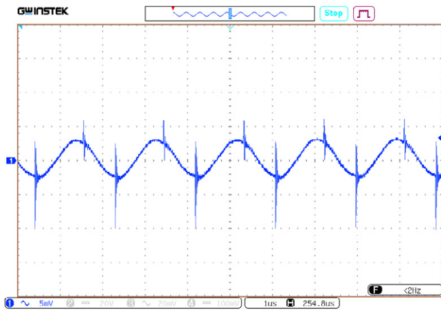
Рис. 57. Осциллограмма пульсаций выходного напряжения.
