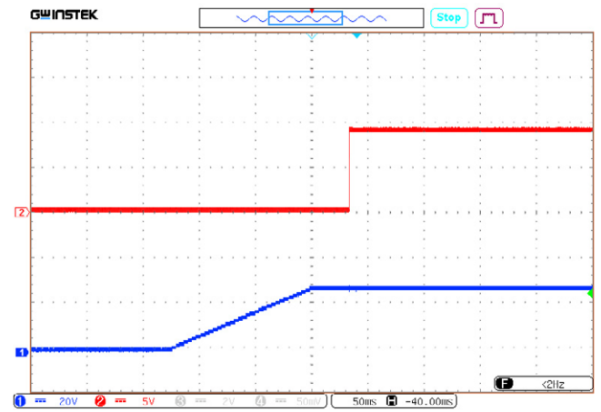
Рис. 56. Осциллограмма установления выходного напряжения с момента подачи входного напряжения.
