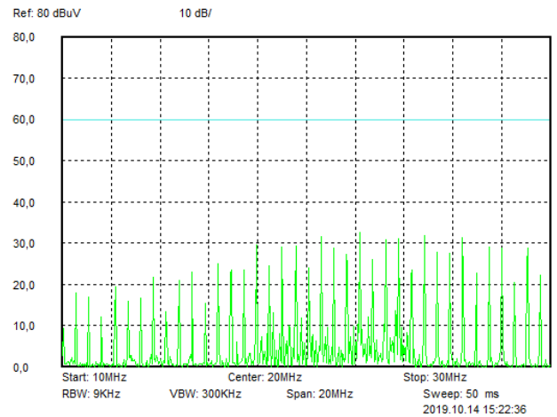
Рис. 66. Диапазон 10..30 МГц.
