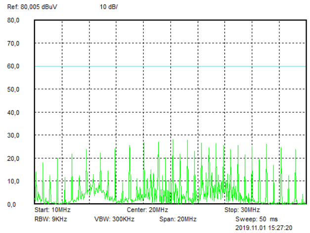
Рис. 68. Диапазон 10..30 МГц.
