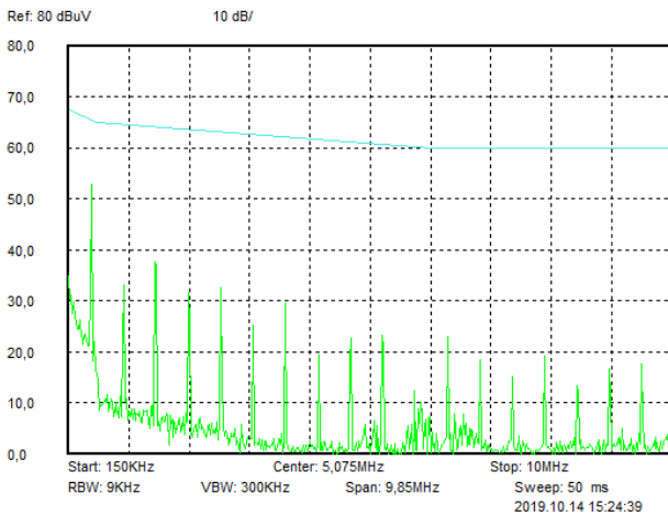
Рис. 65. Диапазон 0,15..10 МГц.
