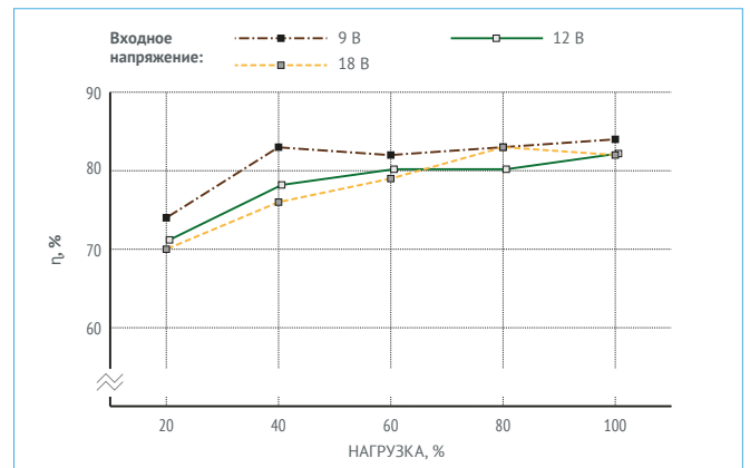
Рис. 22. МДМ10-1А05СР.
