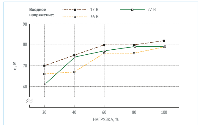
Рис. 18. МДМ6-1В12ТР.
