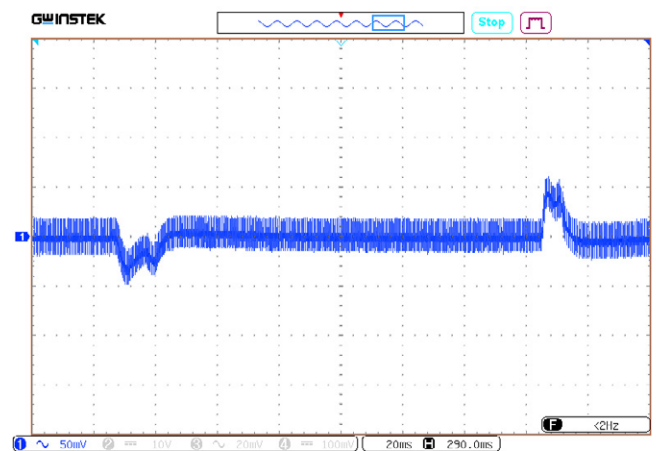
Рис. 50. Осциллограмма переходного отклонения выходного напряжения при изменении выходного тока с 50% до 100%. Масштаб 50 В/дел. Развертка 20 мс/дел.
