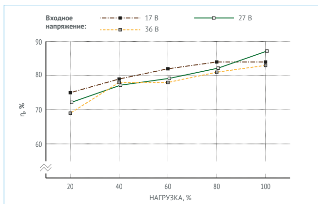
Рис. 30. МДМ10-1В09СР.
