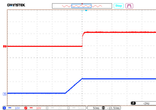
Рис. 52. Осциллограмма установления выходного напряжения с момента подачи входного напряжения.
