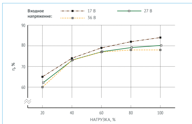
Рис. 19. МДМ6-1В15ТР.
