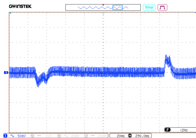
Рис. 50. Осциллограмма переходного отклонения выходного напряжения при изменении выходного тока с 50% до 100 %.
