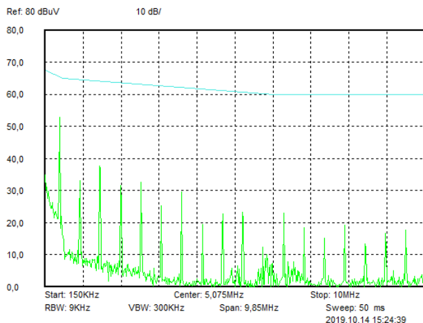
Рис. 65. Диапазон 0,15..10 МГц.
