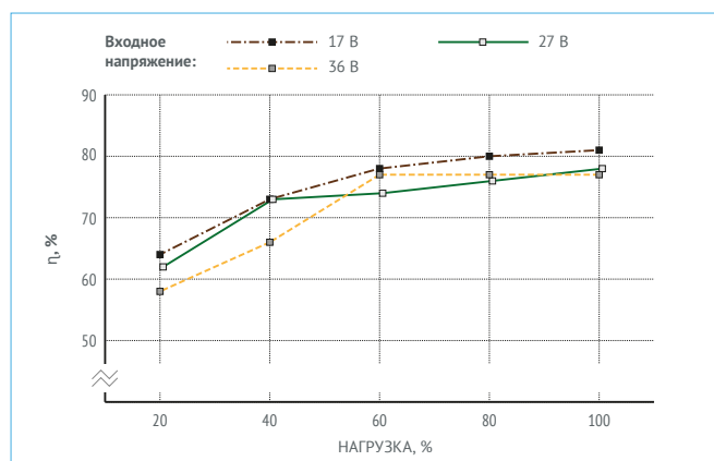
Рис. 16. МДМ6-1B05TP.
