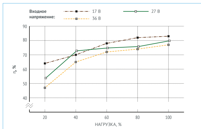
Рис. 20. МДМ6-1В24ТР.
