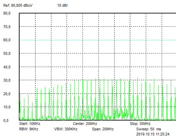
Рис. 72. Диапазон 10..30 МГц.
