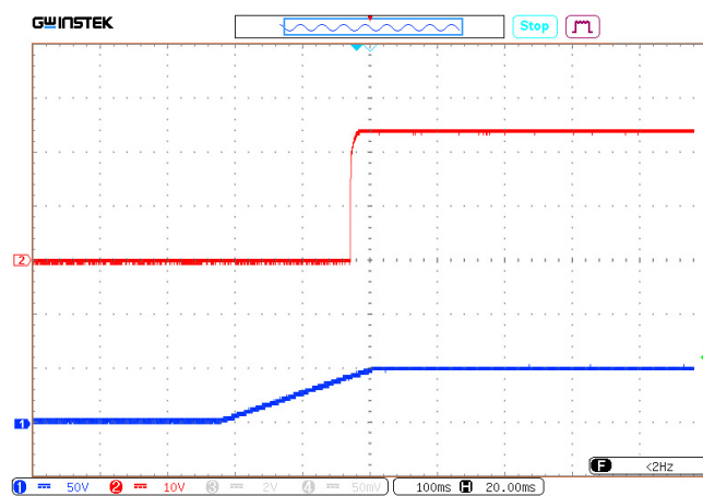
Рис. 60. Осциллограмма установления выходного напряжения с момента подачи входного напряжения. Луч 1 (синий) — входное напряжение. Масштаб 50 В/дел. Луч 2 (красный) — выходное напряжение. Масштаб 10 В/дел. Развертка 100 мс/дел.
