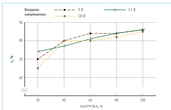
Рис. 27. МДМ10-1A27CP.
