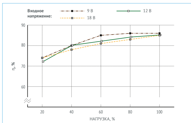
Рис. 23. МДМ10-1A09CP.
