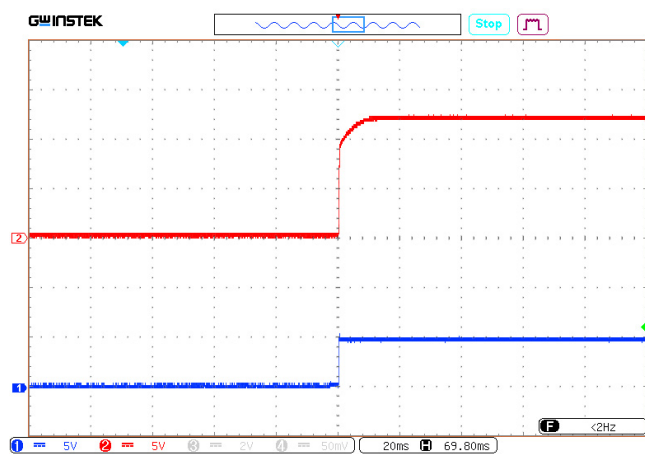
Рис. 47. Осциллограмма установления выходного напряжения с момента подачи команды дистанционного управления.
