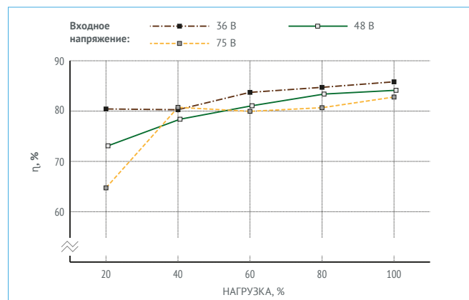
Рис. 35. МДМ10-1Д09СР
