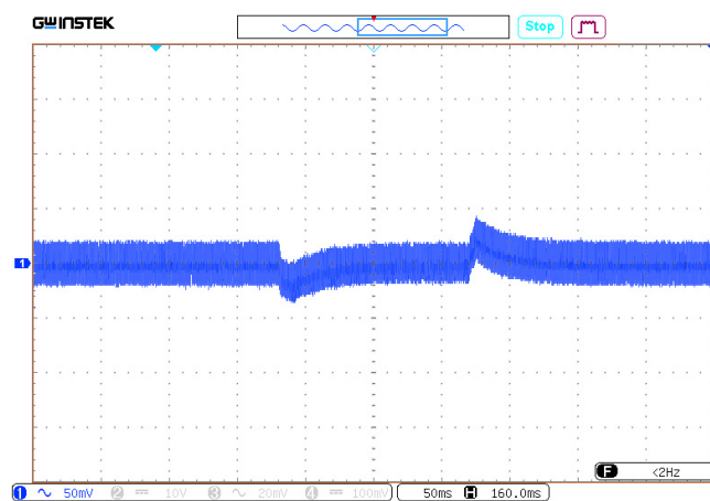
Рис. 58. Осциллограмма переходного отклонения выходного напряжения при изменении выходного тока с 50% до 100 %. Масштаб 50 мВ/дел. Развертка 50 мс/дел.
