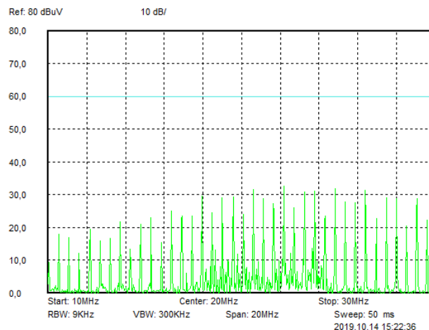
Рис. 66. Диапазон 10..30 МГц.
