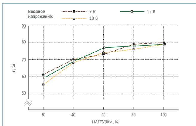
Рис. 8. МДМ6-1А33ТР.
