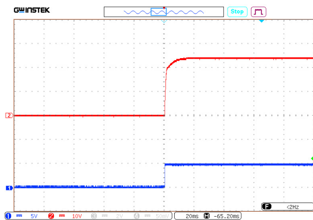
Рис. 59. Осциллограмма установления выходного напряжения с момента подачи команды дистанционного управления. Луч 1 (синий) — напряжение на выходе «ВКЛ». Масштаб 5 В/дел. Луч 2 (красный) — выходное напряжение. Масштаб 10 В/дел. Развертка 20 мс/дел.
