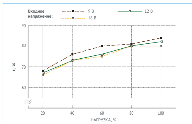
Рис. 9. МДМ6-1А05ТР.
