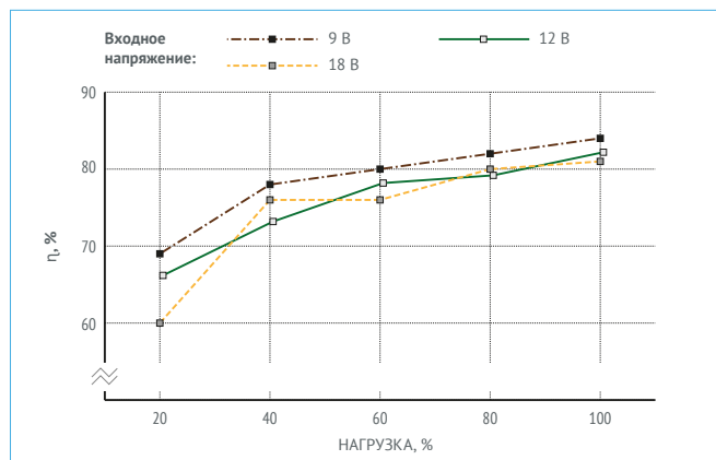
Рис. 11. МДМ6-1А12ТР.
