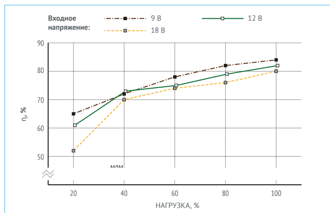
Рис. 14. МДМ6-1A27TP.
