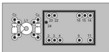
Рис. 3. Вид сверху.
