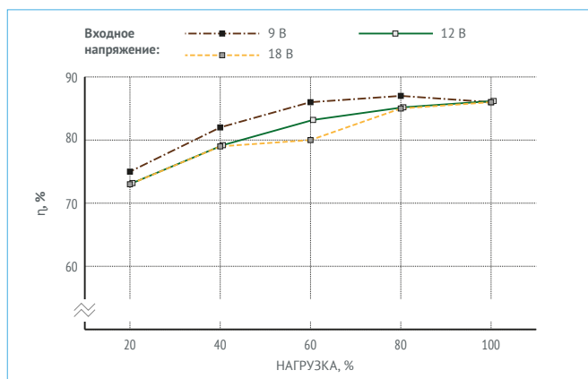
Рис. 25. МДМ10-1A15CP.
