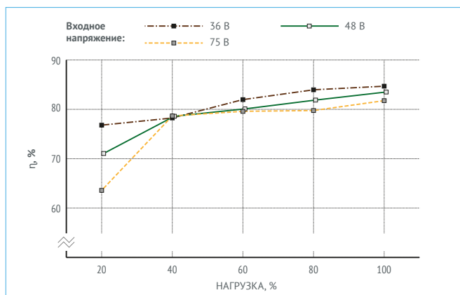
Рис. 36. МДМ10-1Д12СР.
