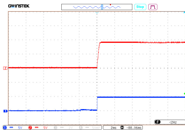
Рис. 55. Осциллограмма установления выходного напряжения с момента подачи команды дистанционного управления. Луч 1 (синий) — напряжение на выводе «ВКЛ». Масштаб 5 В/дел. Луч 2 (красный) — выходное напряжение. Масштаб 5 В/дел. Развертка 2 мс/дел.
