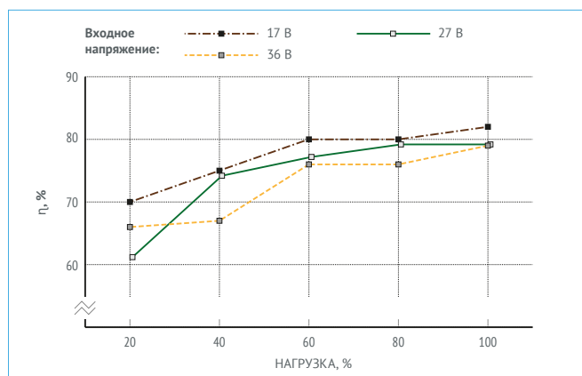
Рис. 18. МДМ6-1В12ТР.
