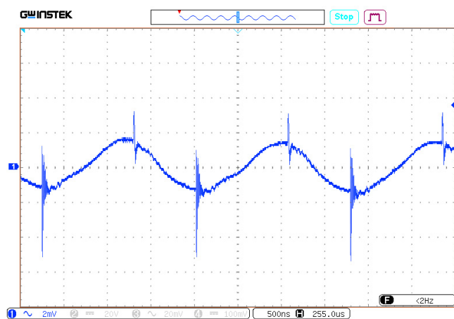
Рис. 53. Осциллограмма пульсаций выходного напряжения.
