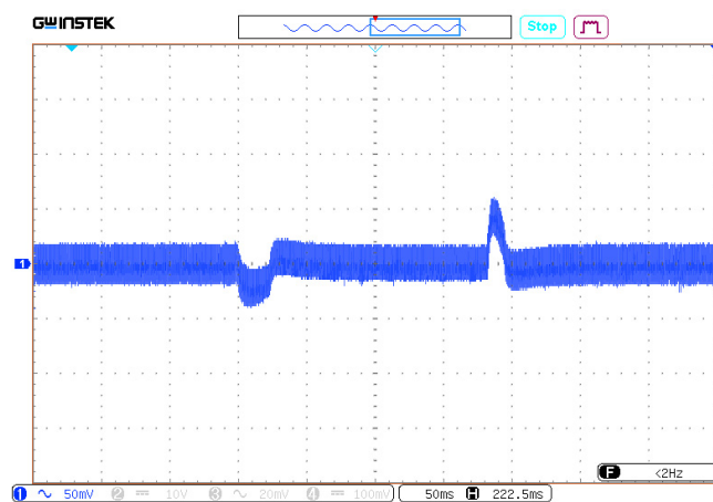
Рис. 62. Осциллограмма переходного отклонения выходного напряжения при изменении выходного тока с 50% до 100 %. Масштаб 50 мВ/дел. Развертка 50 мс/дел.
