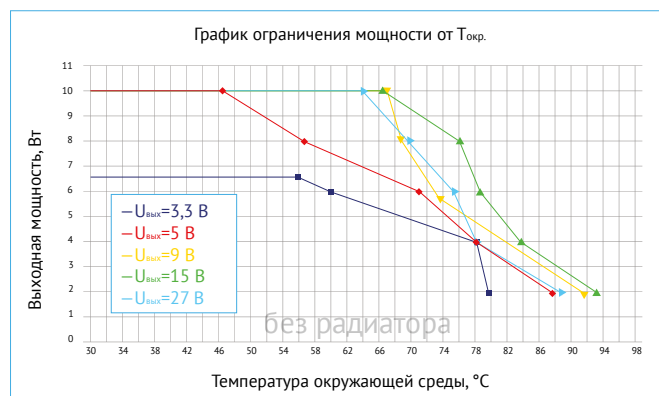
Рис. 41. График ограничения мощности от T_{окр.} без применения внешнего радиатора.
