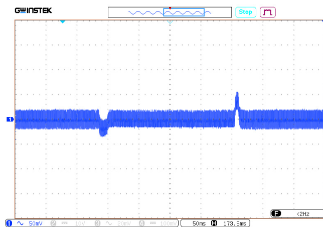
Рис. 54. Осциллограмма переходного отклонения выходного напряжения при изменении выходного тока с 50% до 100 %.
