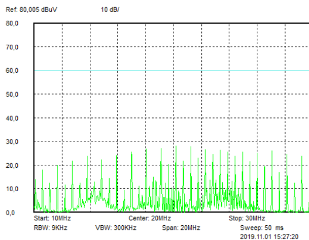
Рис. 68. Диапазон 10..30 МГц.
