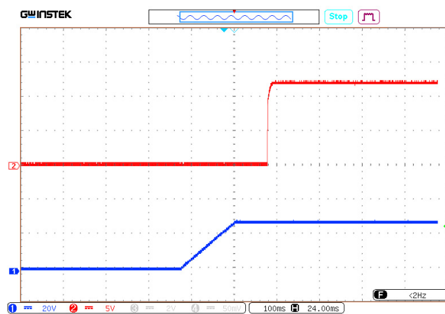
Рис. 48. Осциллограмма установления выходного напряжения с момента подачи входного напряжения.
