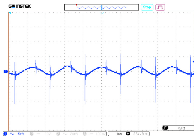
Рис. 49. Осциллограмма пульсаций выходного напряжения.
