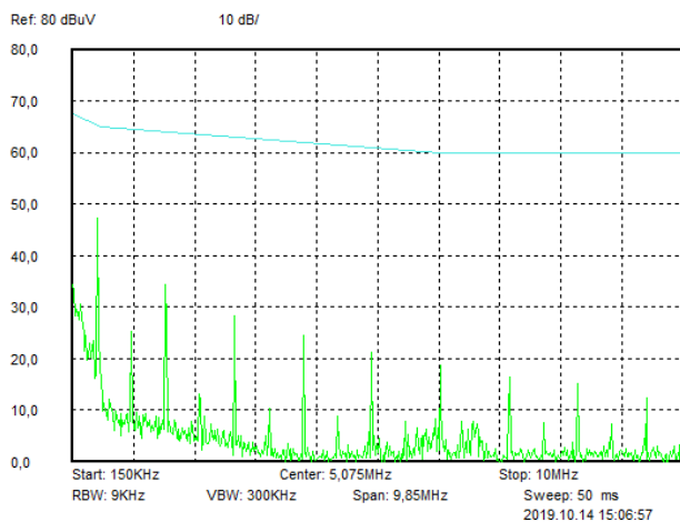
Рис. 63. Диапазон 0,15..10 МГц.
