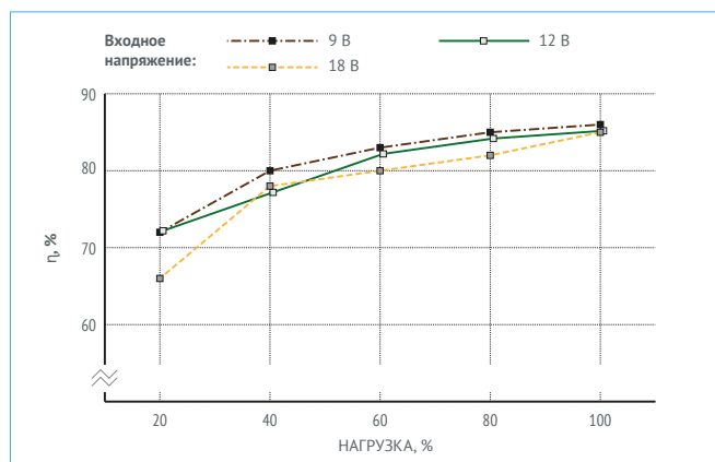
Рис. 26. МДМ10-1A24CP.
