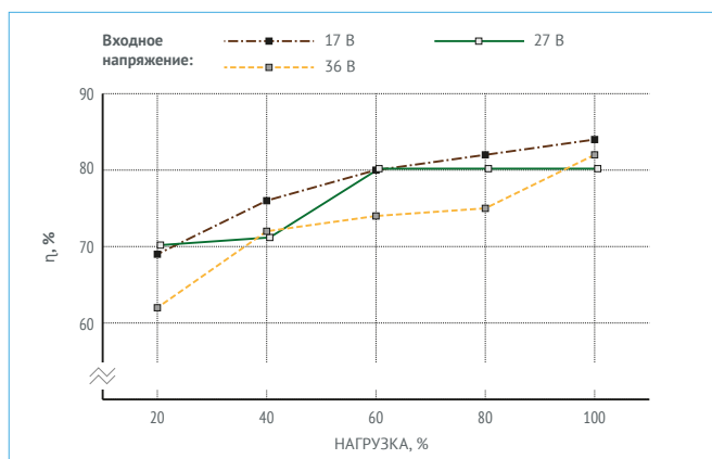
Рис. 17. МДМ6-1В09ТР.
