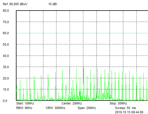
Рис. 70. Диапазон 10..30 МГц.
