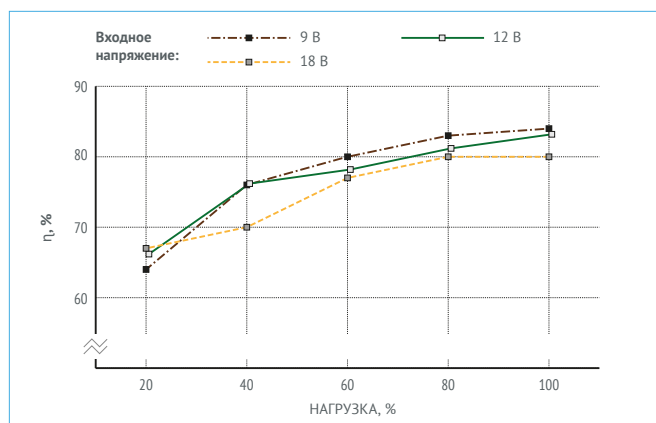
Рис. 12. МДМ6-1A15TP.
