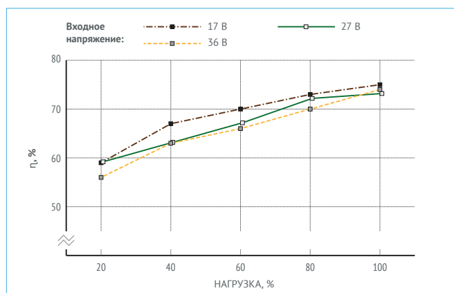
Рис. 15. МДМ6-1B3,3TP.
