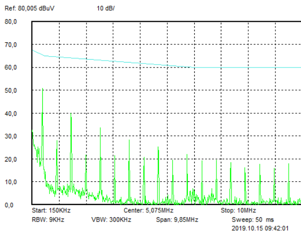
Рис. 69. Диапазон 0,15..10 МГц.
