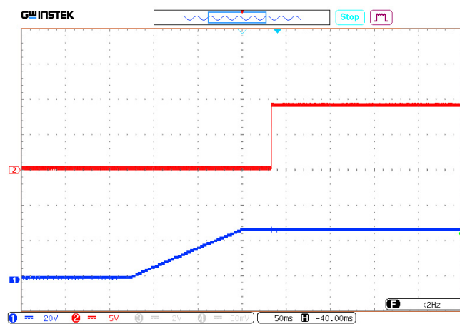
Рис. 56. Осциллограмма установления выходного напряжения с момента подачи входного напряжения. Луч 1 (синий) — входное напряжение. Масштаб 20 В/дел. Луч 2 (красный) — выходное напряжение. Масштаб 5 В/дел. Развертка 50 мс/дел.
