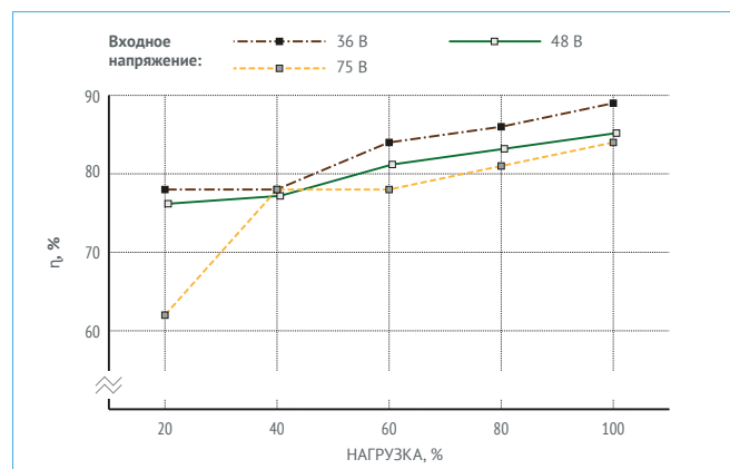
Рис. 37. МДМ10-1Д15СР.
