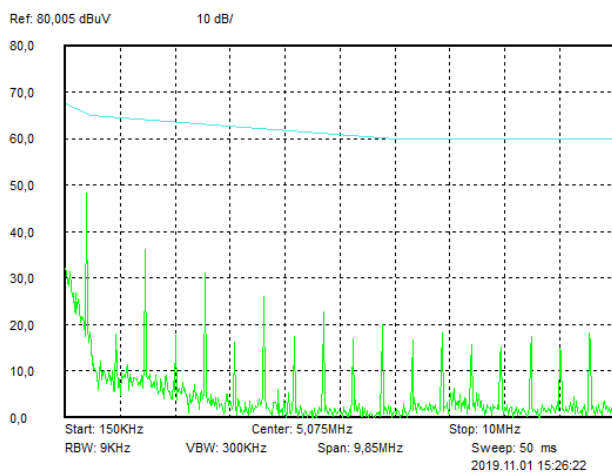
Рис. 67. Диапазон 0,15..10 МГц.
