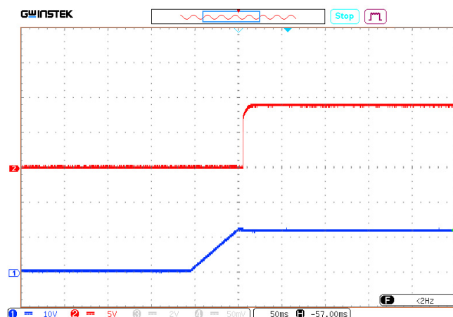
Рис. 44. Осциллограмма установления выходного напряжения с момента подачи входного напряжения.
