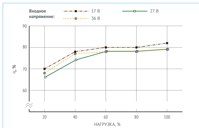
Рис. 29. МДМ10-1В05СР.
