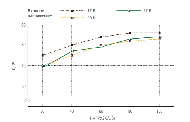
Рис. 31. МДМ10-1В12СР.
