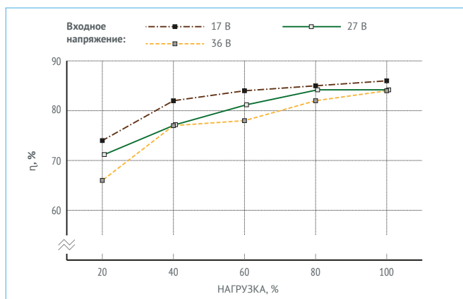
Рис. 32. МДМ10-1В15СР.
