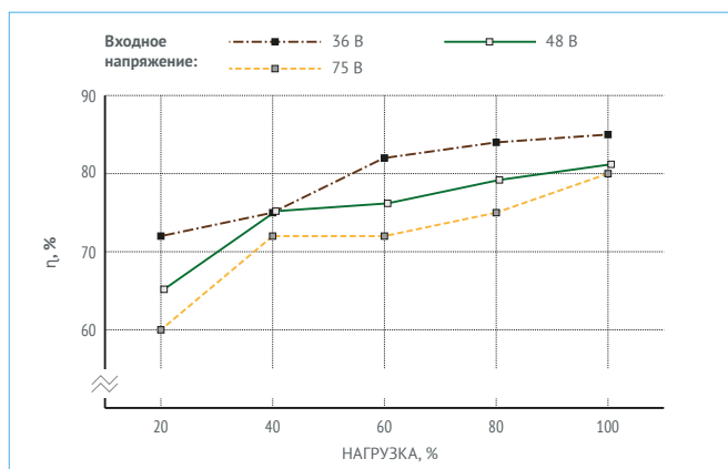
Рис. 38. МДМ10-1Д24СР.
