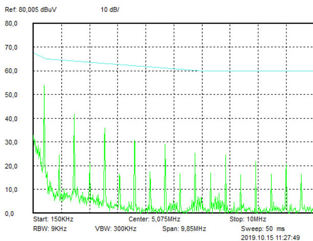
Рис. 71. Диапазон 0,15..10 МГц.
