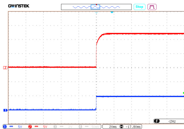
Рис. 51. Осциллограмма установления выходного напряжения с момента подачи команды дистанционного управления.
