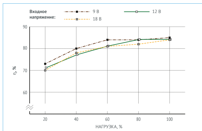
Рис. 24. МДМ10-1A12CP.
