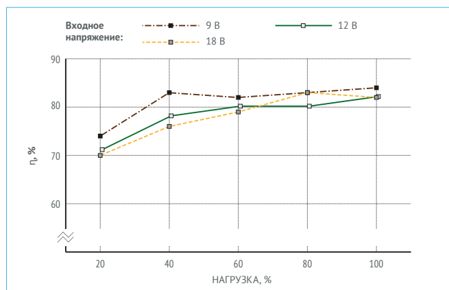
Рис. 22. МДМ10-1А05СР.
