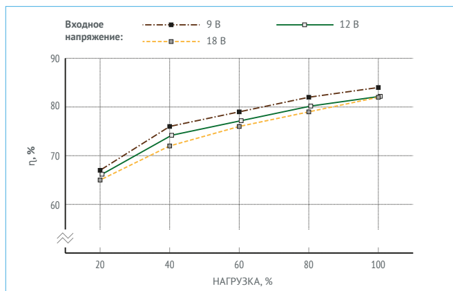
Рис. 10. МДМ6-1А09ТР.
