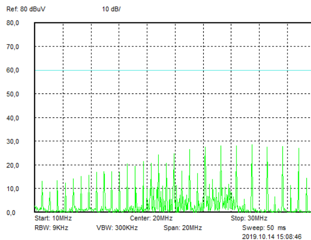
Рис. 64. Диапазон 10..30 МГц.
