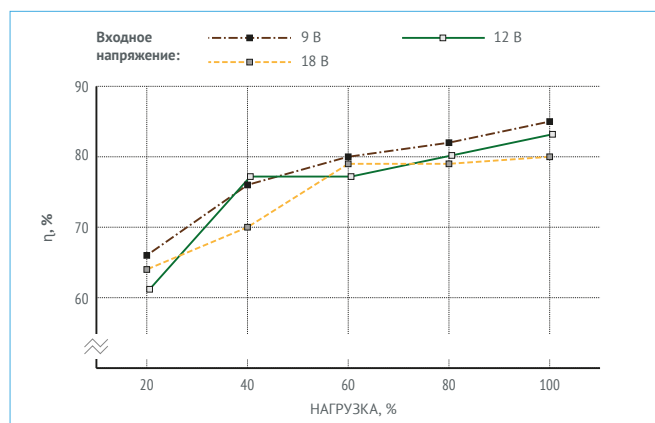
Рис. 13. МДМ6-1A24TP.
