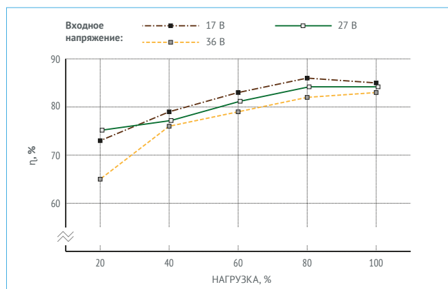
Рис. 33. МДМ10-1В24СР.
