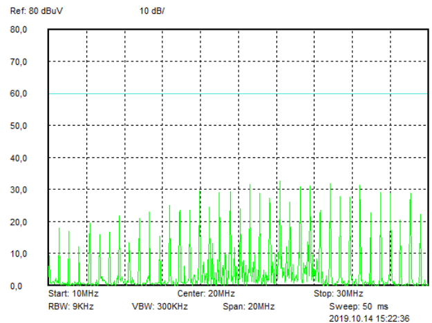
Рис. 66. Диапазон 10..30 МГц.
