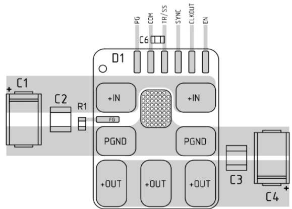
Рис. 4. Рекомендуемая топология печатной платы
