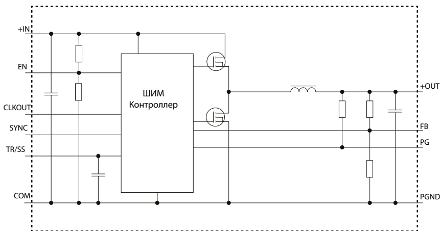
Рис. 2. Функциональная схема модуля электропитания МНМ8
