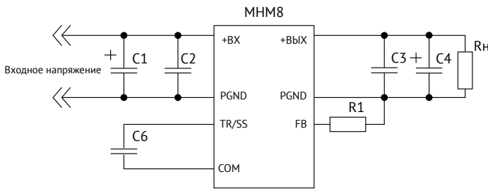
Рис. 3. Типовая схема включения модуля электропитания МНМ
