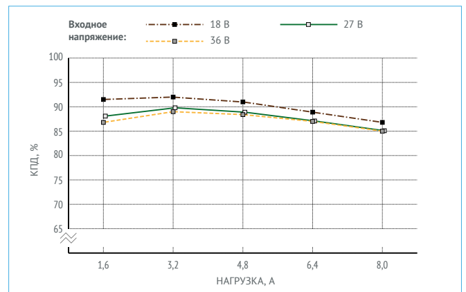
Рис. 13. КПД для МНМ8-1В1,05,0Т. (Выходное напряжение 3,3 В).
