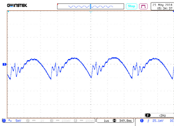
Рис. 25. Осциллограмма пульсаций выходного напряжения модуля Масштаб 5 мВ/дел. Развертка 1 мкс/дел.
