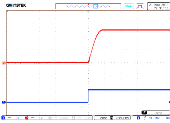
Рис. 21. Осциллограмма установления выходного напряжения с момента подачи команды дистанционного управления.
