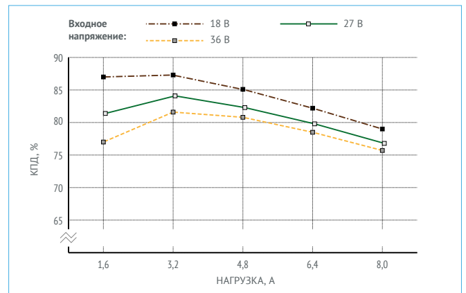
Рис. 11. КПД для МНМ8-1В1,05,0Т. (Выходное напряжение 1,8 В).
