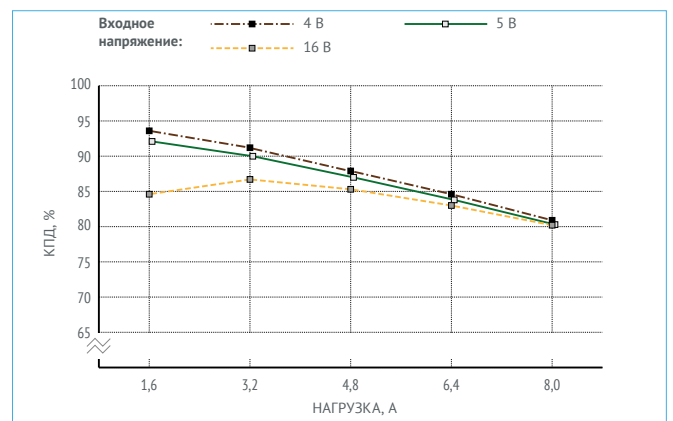
Рис. 18. КПД для МНМ8-1И1,05,0Т. (Выходное напряжение 1,8 В).
