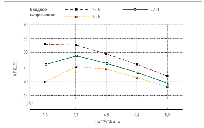
Рис. 9. КПД для МНМ8-1В1,05,0Т. (Выходное напряжение 1,2 В).
