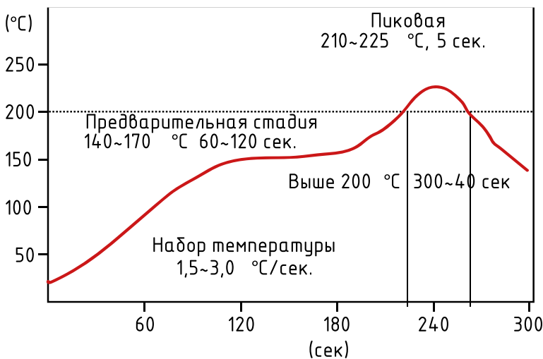
Рис. 5. Профиль оплавления
