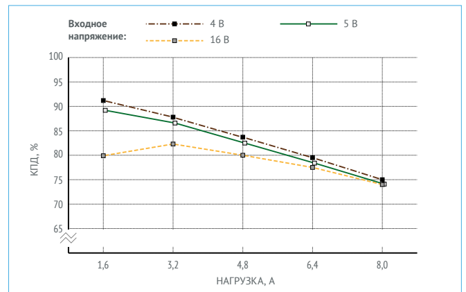
Рис. 16. КПД для МНМ8-1И1,05,0Т. (Выходное напряжение 1,2 В).
