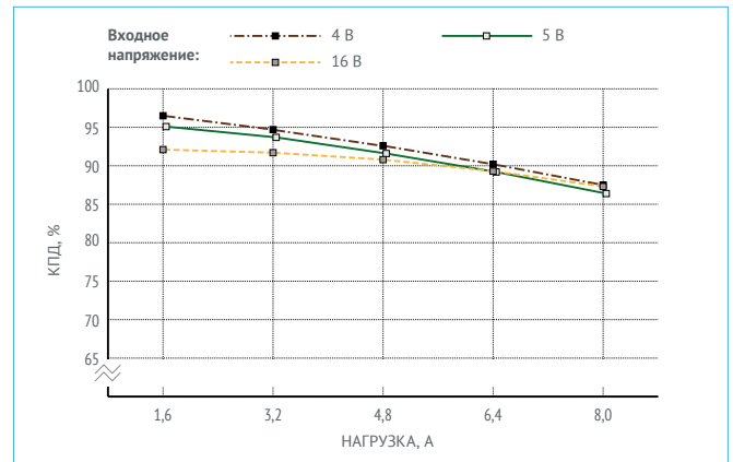
Рис. 20. КПД для МНМ8-1И1,05,0Т. (Выходное напряжение 3,3 В).
