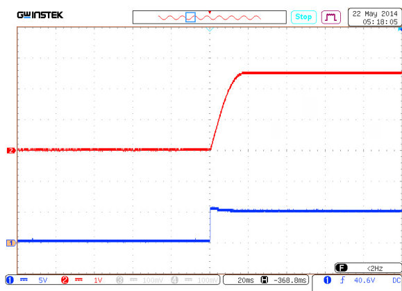
Рис. 26. Осциллограмма установления выходного напряжения с момента подачи команды дистанционного управления. Луч 1 (синий) — напряжение на выводе «EN». Масштаб 5 В/дел. Луч 2 (красный) — выходное напряжение. Масштаб 1 В/дел. Развертка 20 мс/дел.
