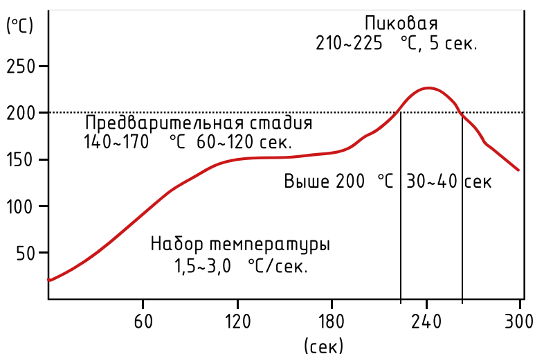
Рис. 5. Профиль оплавления
