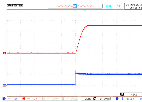
Рис. 27. Осциллограмма установления выходного напряжения с момента подачи входного напряжения. Луч 1 (синий) — входное напряжение. Масштаб 5 В/дел. Луч 2 (красный) — выходное напряжение. Масштаб 1 В/дел. Развертка 20 мс/дел.
