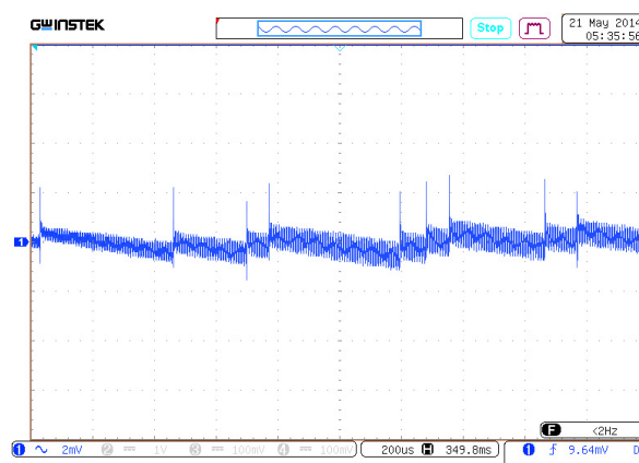
Рис. 24. Осциллограмма пульсаций выходного напряжения модуля в режиме пропуска импульсов.
