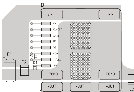
Рис. 4. Рекомендуемая топология печатной платы
