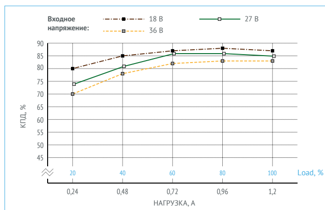
Рис. 11. КПД для МНМ1,2-1В1,05,0Т. (Выходное напряжение 2 В).
