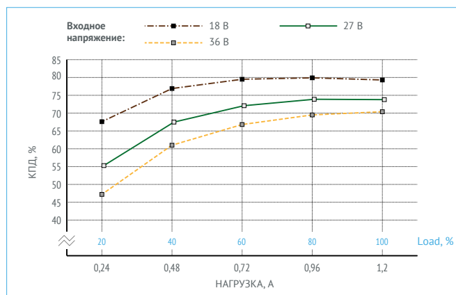
Рис. 9. КПД для МНМ1,2-1В1,05,0Т. (Выходное напряжение 1,2 В).
