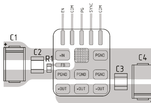
Рис. 4. Рекомендуемая топология печатной платы
