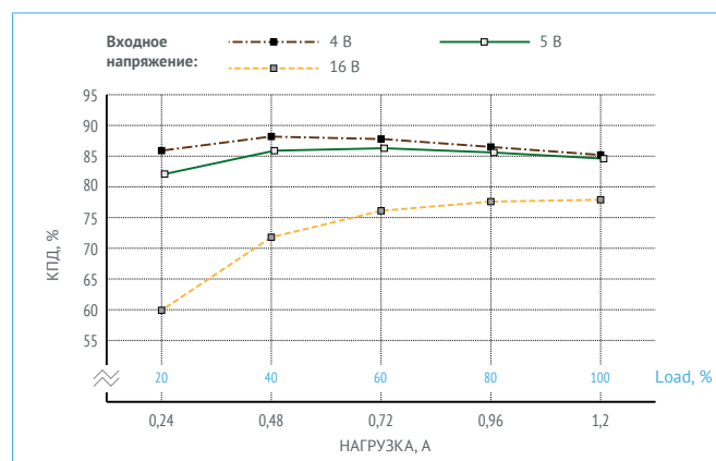
Рис. 16. КПД для МНМ1,2-1И1,05,0Т. (Выходное напряжение 1,2 В).
