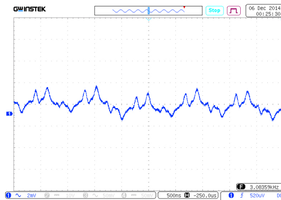
Рис. 29. Осциллограмма пульсаций выходного напряжения.
