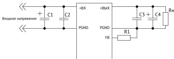
Рис. 3. Типовая схема включения модуля электропитания МНМ
