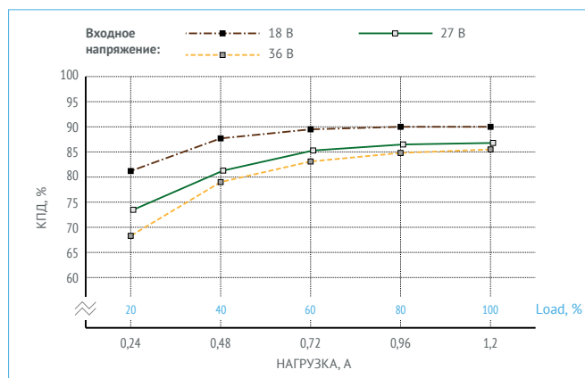
Рис. 13. КПД для МНМ1,2-1В1,05,0Т. (Выходное напряжение 3,3 В).
