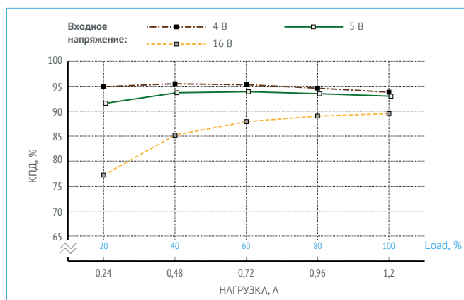
Рис. 20. КПД для МНМ1,2-1И1,05,0Т. (Выходное напряжение 3,3 В).
