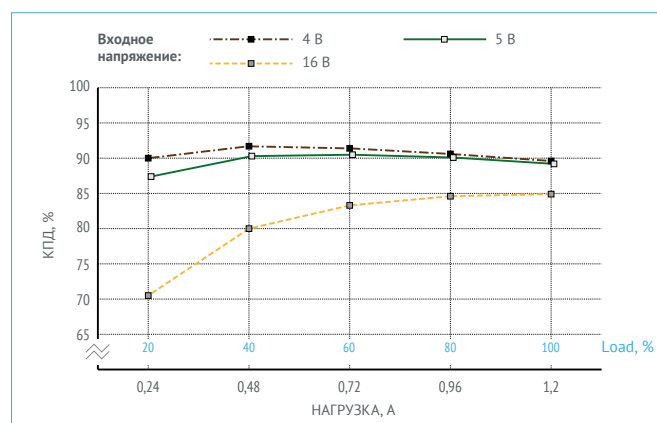
Рис. 18. КПД для МНМ1,2-1И1,05,0Т. (Выходное напряжение 2 В).
