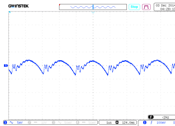
Рис. 25. Осциллограмма пульсаций выходного напряжения.
