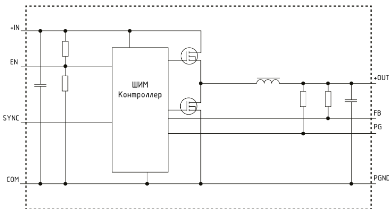
Рис. 2. Функциональная схема модуля электропитания МНМ1,2
