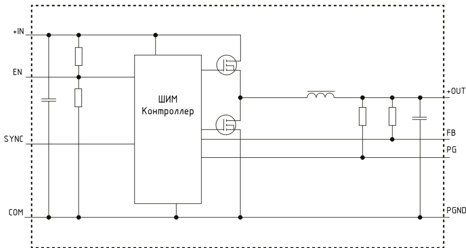
Рис. 2. Функциональная схема модуля электропитания МНМ1,2.
