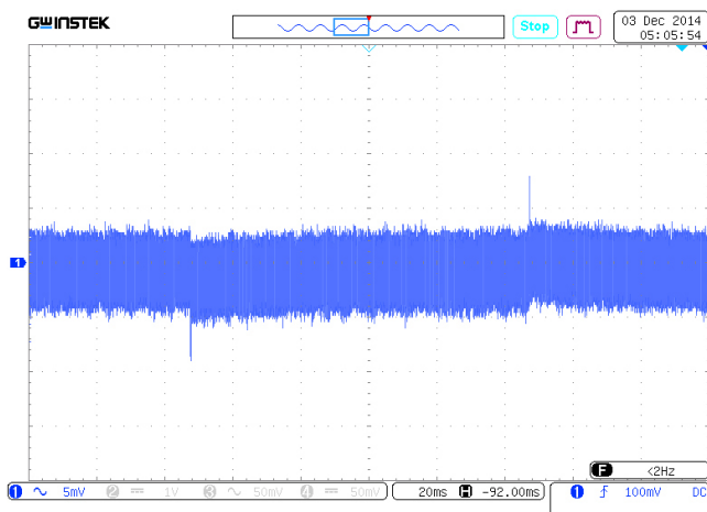
Рис. 28. Осциллограмма переходного отклонения выходного напряжения при изменении выходного тока на 25%. Масштаб 5 мВ/дел. Развертка 20 мс/дел.
