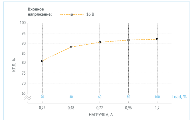
Рис. 21. КПД для МНМ1,2-1И1,05,0Т. (Выходное напряжение 5 В).
