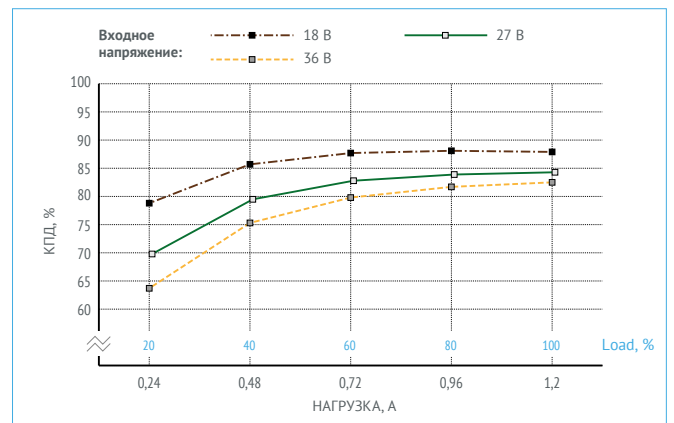
Рис. 12. КПД для МНМ1,2-1В1,05,0Т. (Выходное напряжение 2,5 В).
