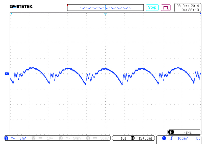
Рис. 29. Осциллограмма пульсаций выходного напряжения. Масштаб 2 мВ/дел. Развертка 500 нс/дел.
