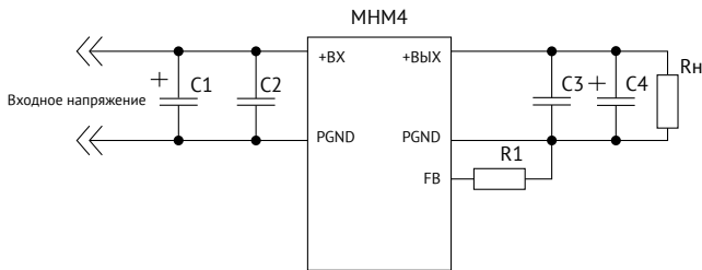
Рис. 3. Типовая схема включения модуля электропитания МНМ.
