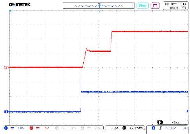
Рис. 27. Осциллограмма установления выходного напряжения с момента подачи входного напряжения. Луч 1 (синий) – входное напряжение. Масштаб 5 В/дел. Луч 2 (красный) – выходное напряжение. Масштаб 2 В/дел. Развертка 5 мс/дел.
