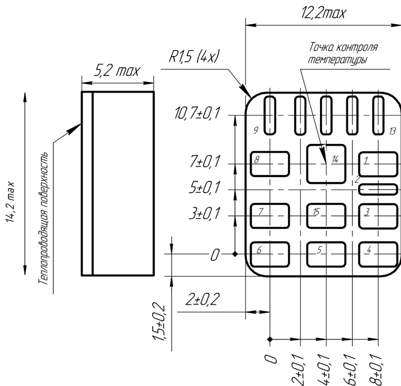
Рис. 30. Габаритный чертёж, вид снизу.
