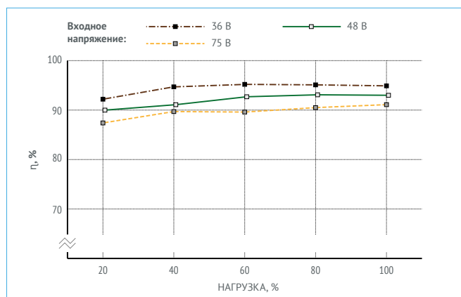
Рис. 23. МДМ500-1Д24ТУР.
