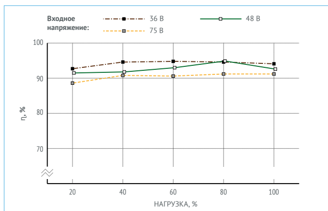
Рис. 22. МДМ500-1Д15ТУР.
