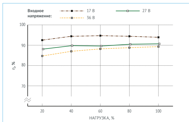
Рис. 19. МДМ500-1В27ТУР.
