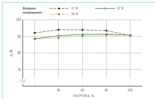
Рис. 16. МДМ500-1В12ТУР.
