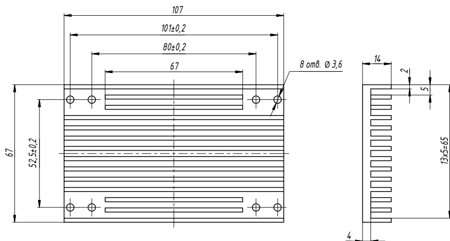
Рис. 38. БКЯЮ.752695.265.
