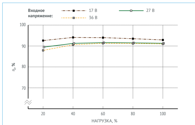
Рис. 15. МДМ500-1В09ТУР.
