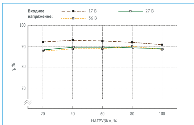
Рис. 17. МДМ500-1В15ТУР.
