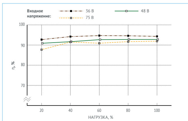
Рис. 20. МДМ500-1Д09ТУР.
