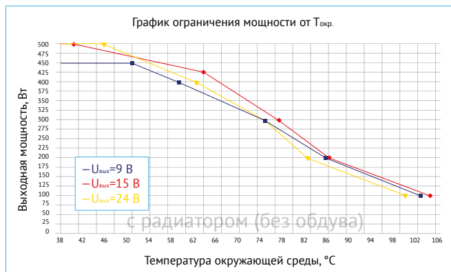
Рис. 26. График ограничения мощности от T_{ОКР.} с применением внешнего радиатора БКЯЮ.752695.265-01 ( S=631 \text{ см}^2 ) без принудительного обдува.
