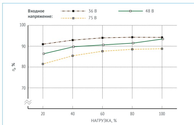
Рис. 24. МДМ500-1Д27ТУР.
