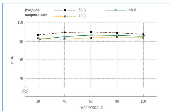
Рис. 21. МДМ500-1Д12ТУР.
