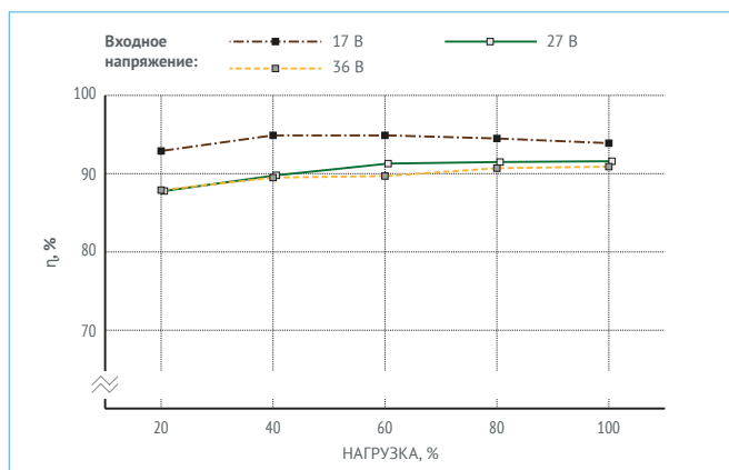
Рис. 18. МДМ500-1В24ТУР.
