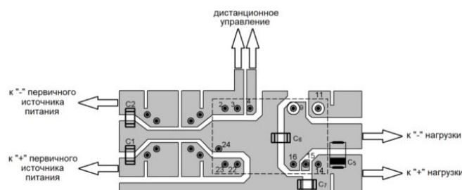
Рис. 4. Вид снизу.
