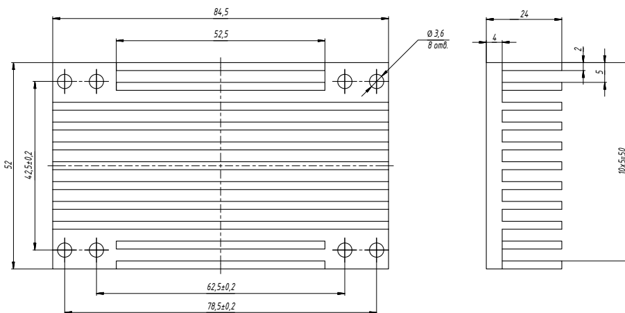
Рис. 39. БКЯЮ.752695.264-01.
