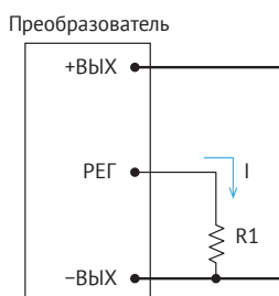
Рис. 8. Увеличение U_{вых} .
