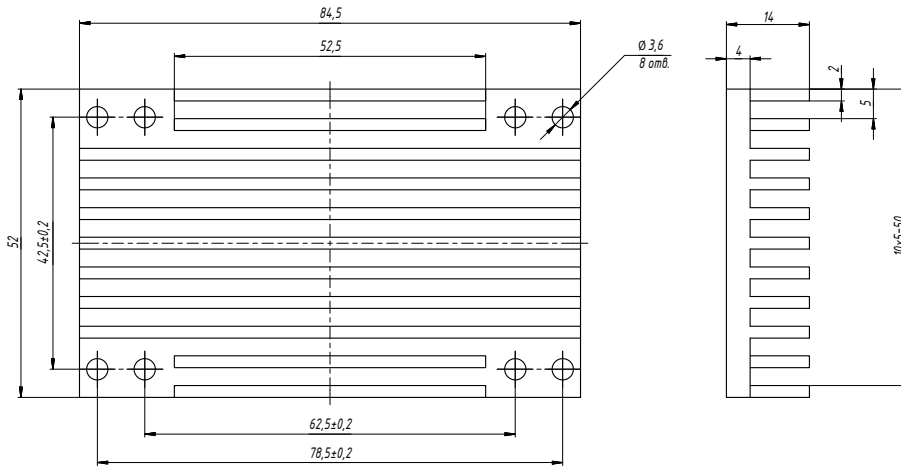
Рис. 38. БКЯЮ.752695.264.
