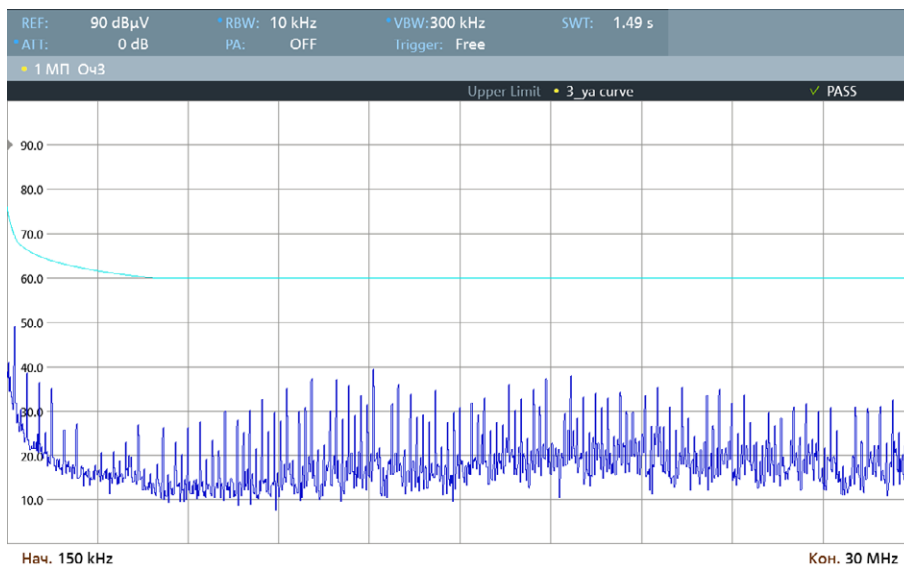
Рис. 36. Диапазон 0,15..30 МГц.
