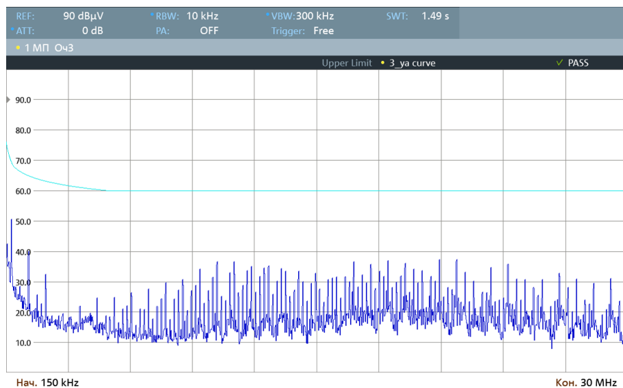
Рис. 35. Диапазон 0,15..30 МГц.
