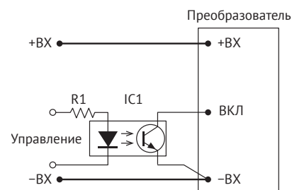
Рис. 7. ВКЛ/ВЫКЛ с помощью оптрона.
