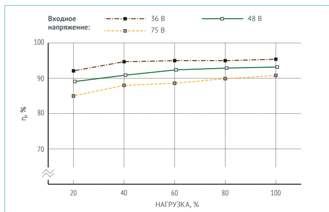
Рис. 23. МДМ300-1Д24ТУР.
