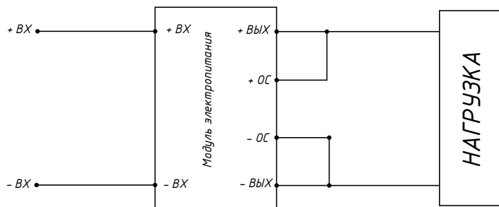
Рис. 14. Схема включения выносной ОС в случае, когда функция выносной ОС не используется.
