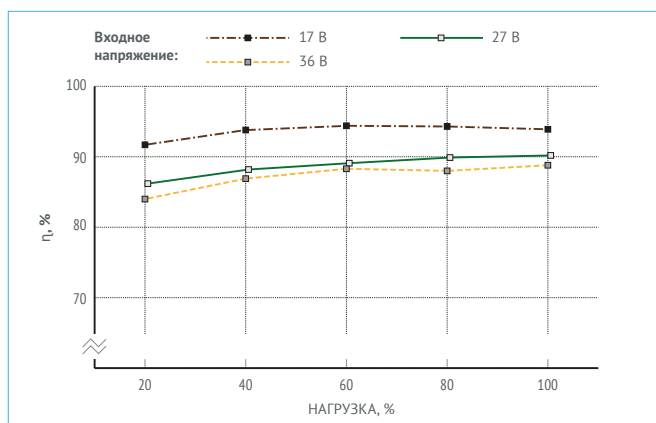
Рис. 19. МДМ300-1В27ТУР.
