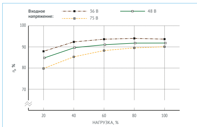
Рис. 22. МДМ300-1Д15ТУР.
