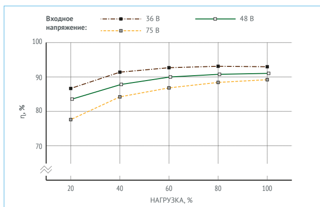
Рис. 20. МДМ300-1Д09ТУР.
