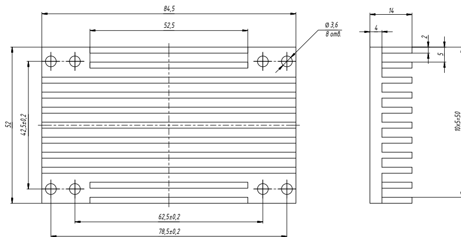
Рис. 38. БКЯЮ.752695.264.
