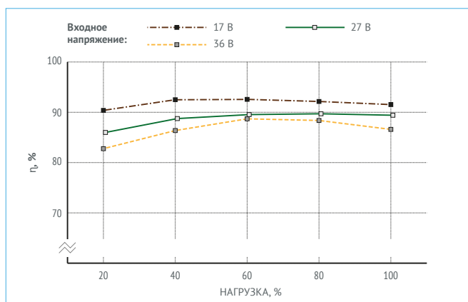
Рис. 15. МДМ300-1В09ТУР.
