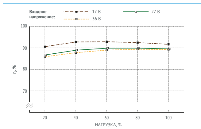
Рис. 16. МДМ300-1В12ТУР.
