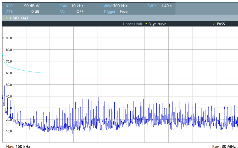
Рис. 36. Диапазон 0,15..30 МГц.
