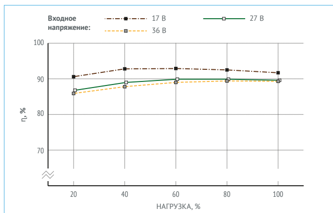
Рис. 17. МДМ300-1В15ТУР.
