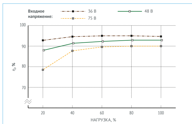
Рис. 21. МДМ300-1Д12ТУР.
