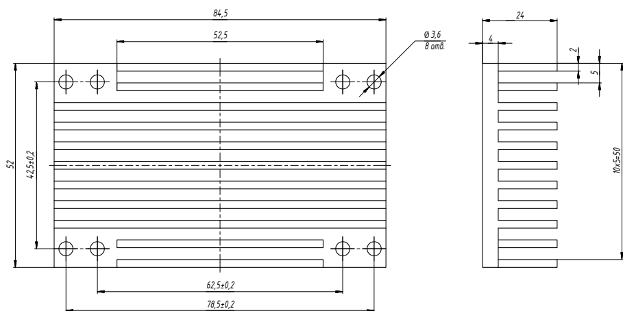
Рис. 39. БКЯЮ.752695.264-01.
