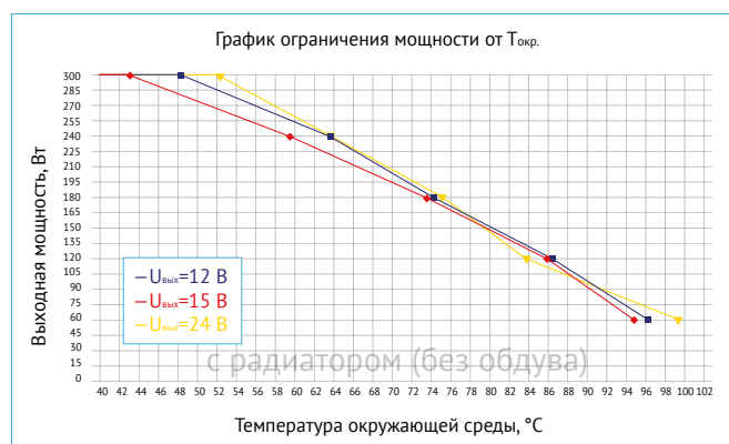
Рис. 26. График ограничения мощности от T_{ОКР} с применением внешнего радиатора БКЯЮ.752695.264-01 ( S=383 \text{ см}^2 ) без принудительного обдува.
