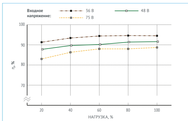
Рис. 24. МДМ300-1Д27ТУР.
