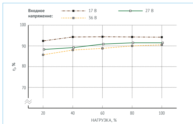
Рис. 18. МДМ300-1В24ТУР.
