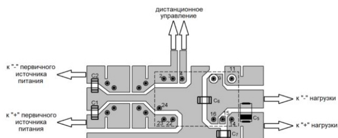
Рис. 4. Вид снизу.
