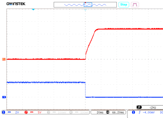
Рис. 27. Осциллограмма установления выходного напряжения с момента подачи команды дистанционного управления. Луч 1 (синий) – напряжение на выводе «VKЛ». Масштаб 2 В/дел. Луч 2 (красный) – выходное напряжение. Масштаб 5 В/дел. Развертка 20 мс/дел.
