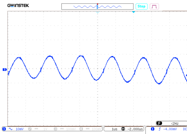
Рис. 25. Осциллограмма пульсаций выходного напряжения.
