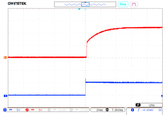
Рис. 24. Осциллограмма установления выходного напряжения с момента подачи входного напряжения.
