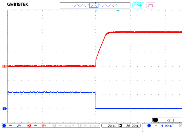
Рис. 31. Осциллограмма установления выходного напряжения с момента подачи команды дистанционного управления. Луч 1 (синий) – напряжение на выводе «ВКЛ». Масштаб 2 В/дел. Луч 2 (красный) – выходное напряжение. Масштаб 5 В/дел. Развертка 20 мс/дел.
