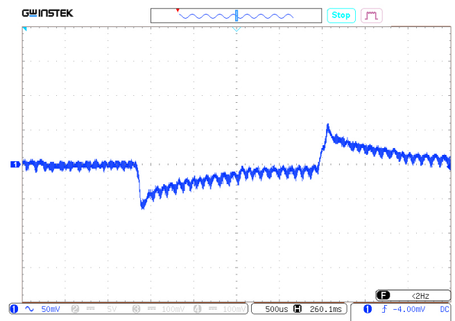
Рис. 26. Осциллограмма переходного отклонения выходного напряжения при изменении выходного тока.
