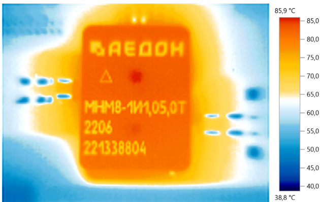
Рис. 33. Верхняя сторона. 85,9 °C
