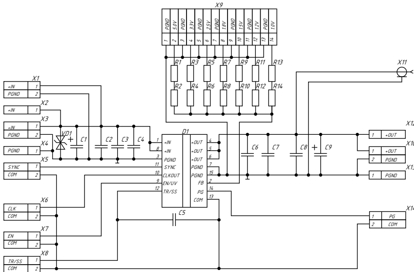
Рис. 3. Принципиальная электрическая схема демоплат МНМ8-ДП-1И1,05,0; МНМ8-ДП-1В1,05,0.
