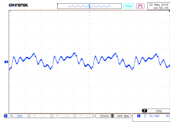
Рис. 14. Осциллограмма пульсаций выходного напряжения модуля при I_{OUT} = 8\text{ A} . Масштаб 2 мВ/дел. Развертка 500 нс/дел.
