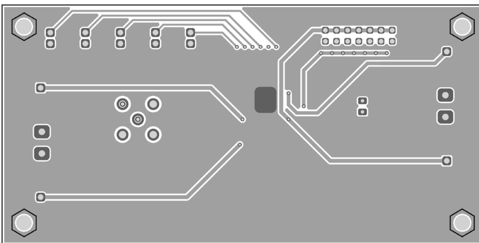
Рис. 5. Нижняя сторона.
