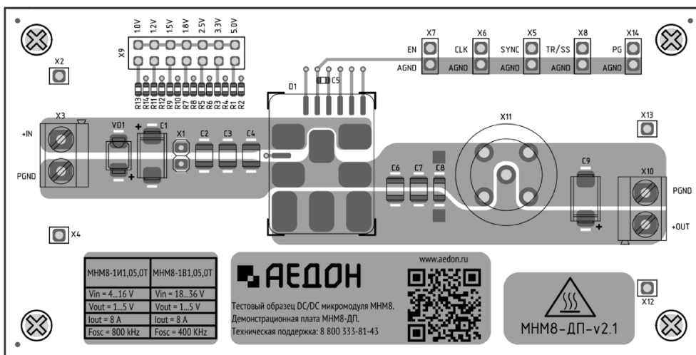
Рис. 4. Верхняя сторона.
