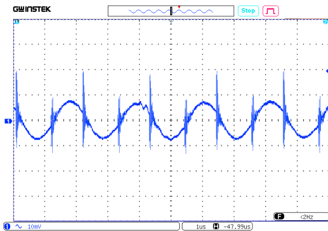
Рис. 22. Осциллограмма пульсаций выходного напряжения.
