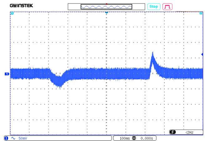
Рис. 23. Осциллограмма переходного отклонения выходного напряжения при изменении выходного тока на 50%.
