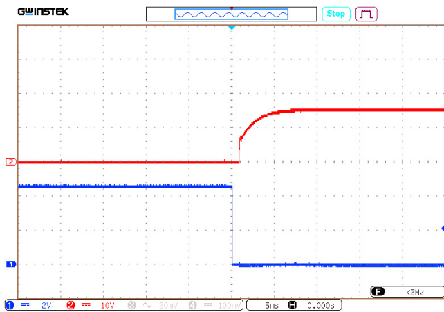
Рис. 24. Осциллограмма установления выходного напряжения с момента подачи команды дистанционного управления. Луч 1 (синий) – напряжение на выводе «VKЛ». Масштаб 2 В/дел. Луч 2 (красный) – выходное напряжение. Масштаб 10 В/дел. Развертка 5 мс/дел.
