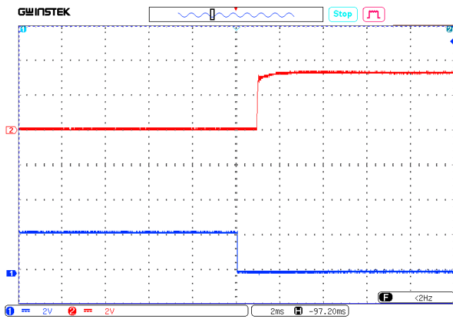
Рис. 20. Осциллограмма установления выходного напряжения с момента подачи команды дистанционного управления.
