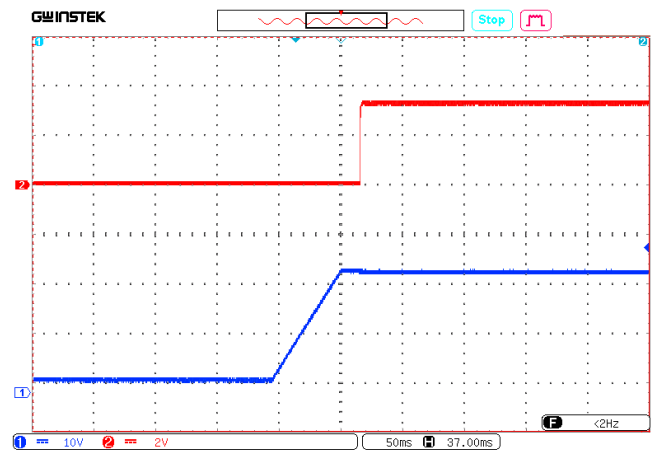
Рис. 21. Осциллограмма установления выходного напряжения с момента подачи входного напряжения.
