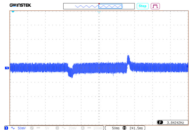
Рис. 19. Осциллограмма переходного отклонения выходного напряжения при изменении выходного тока на 50%.
