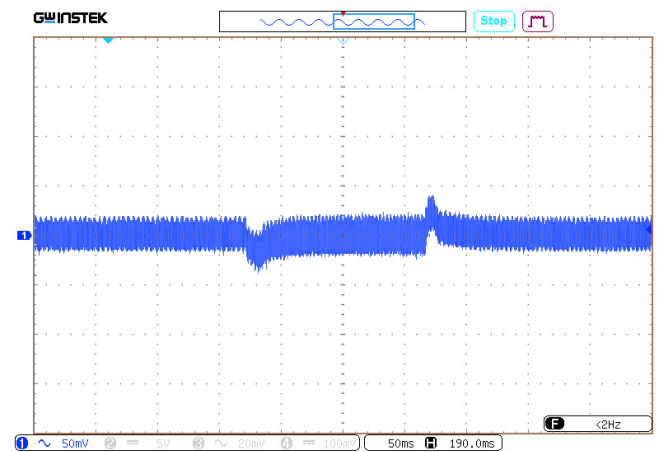
Рис. 27. Осциллограмма переходного отклонения выходного напряжения при изменении выходного тока. Масштаб 50 мВ/дел. Развертка 50 мс/дел.
