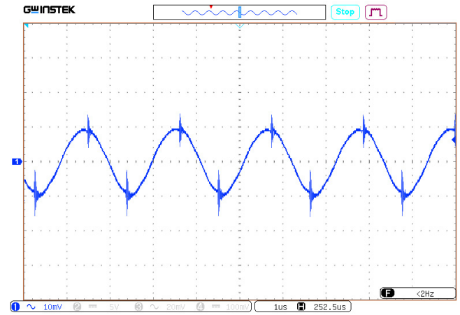
Рис. 18. Осциллограмма пульсации выходного напряжения.
