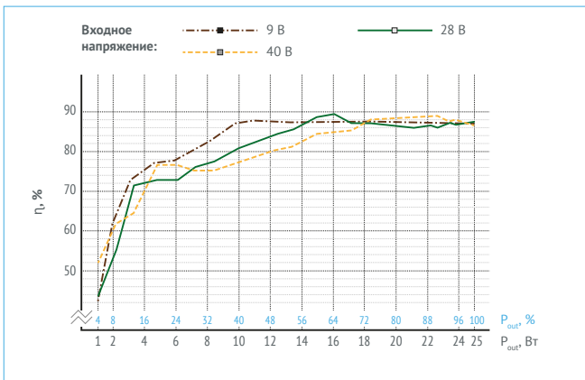
Рис. 15. МДМ25-1Б15РС.
