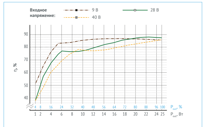
Рис. 16. МДМ25-1Б28РС.
