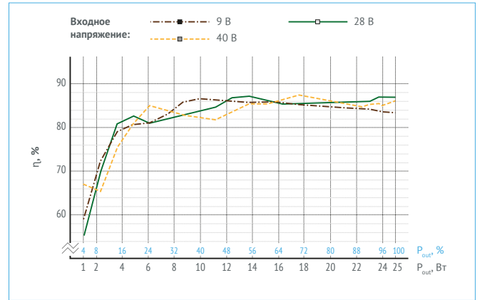
Рис. 12. МДМ25-1Б05РС.
