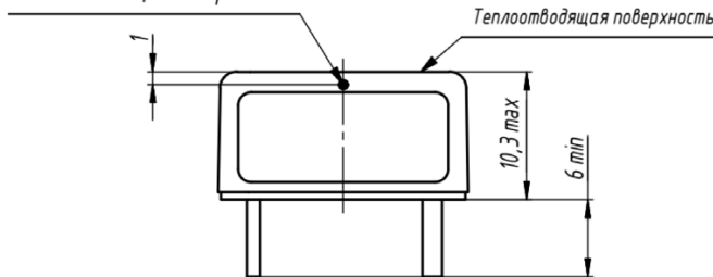
Рис. 18. Исполнение МДМ25-С.
