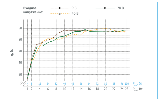
Рис. 14. МДМ25-1Б12РС.
