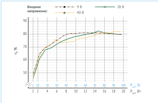
Рис. 11. МДМ25-1Б3,3РС.
