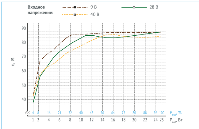
Рис. 17. МДМ25-1Б48РС.
