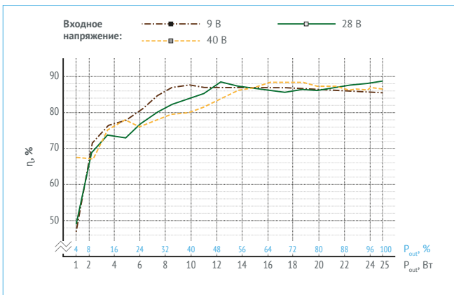
Рис. 13. МДМ25-1Б09РС.
