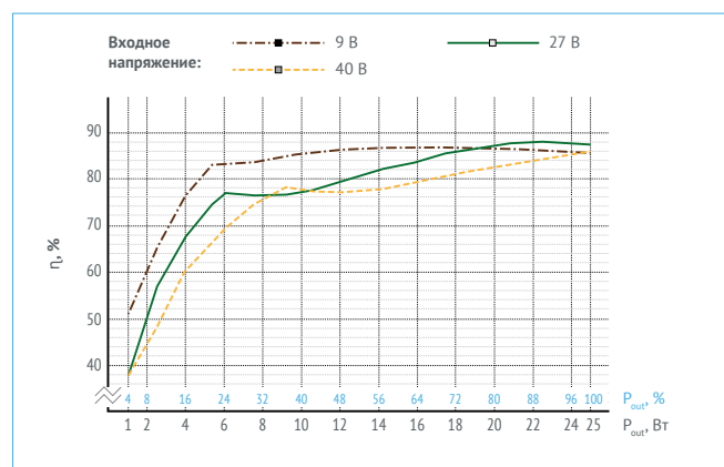
Рис. 16. МДМ25-1Б27РС.
