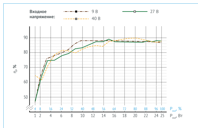
Рис. 14. МДМ25-1Б12РС.
