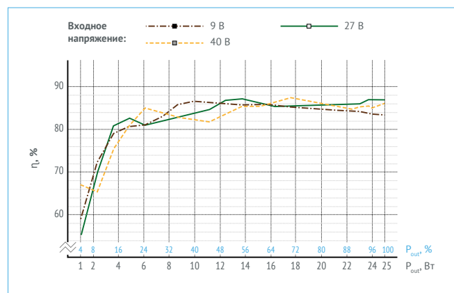
Рис. 12. МДМ25-1Б05РС.
