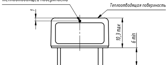
Рис. 18. Исполнение МДМ25-С.
