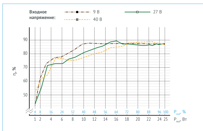
Рис. 15. МДМ25-1Б15РС.
