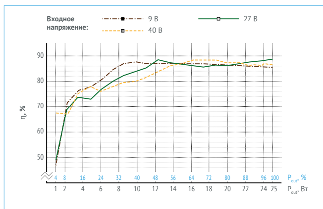
Рис. 13. МДМ25-1Б09РС.
