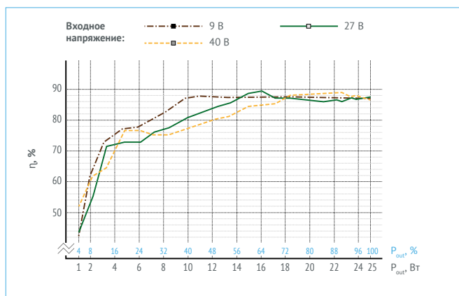
Рис. 15. МДМ25-1B15PC.
