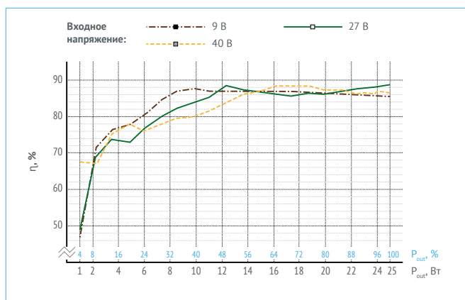
Рис. 13. МДМ25-1B09PC.
