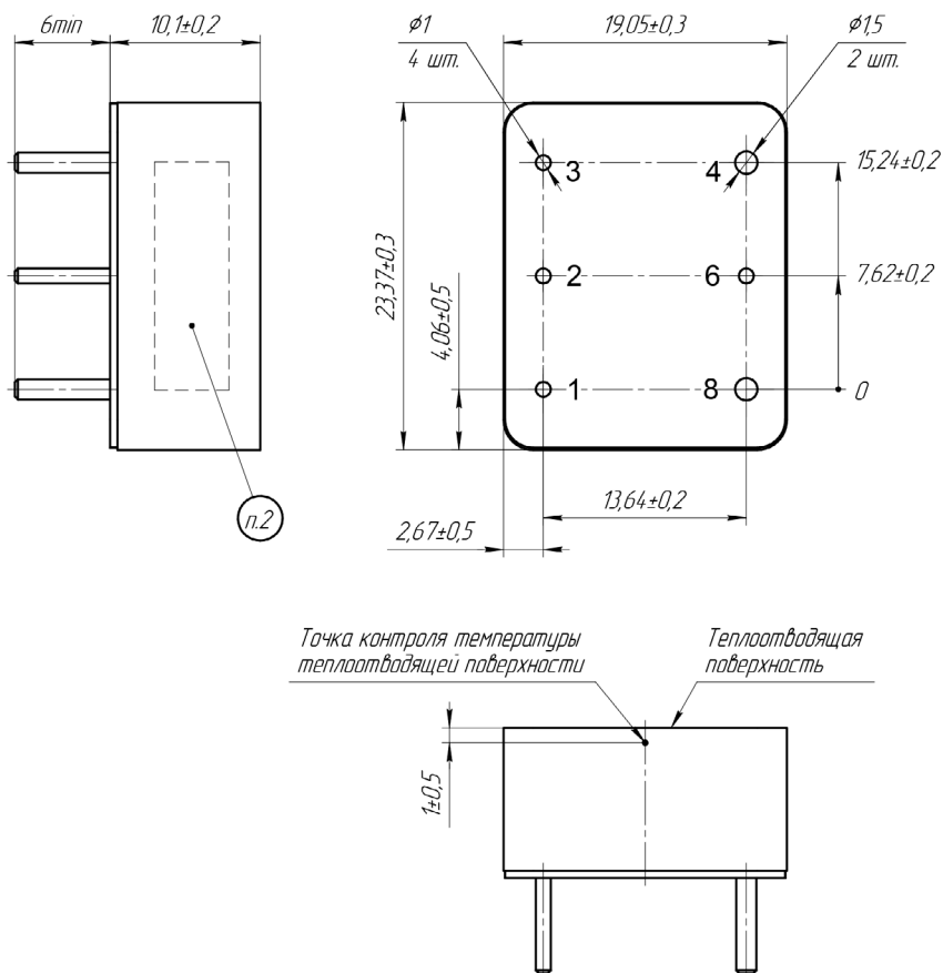
Рис. 18. Исполнение МДМ25-С.
