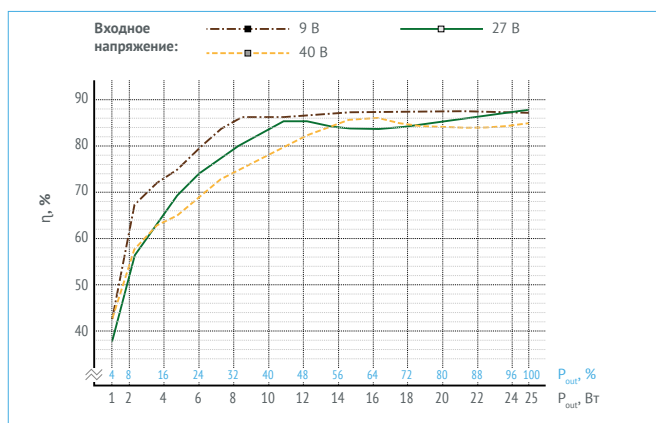
Рис. 17. МДМ25-1B48PC.
