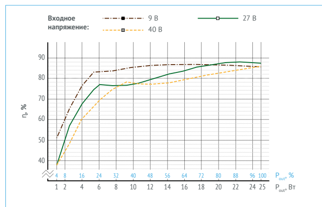
Рис. 16. МДМ25-1B27PC.
