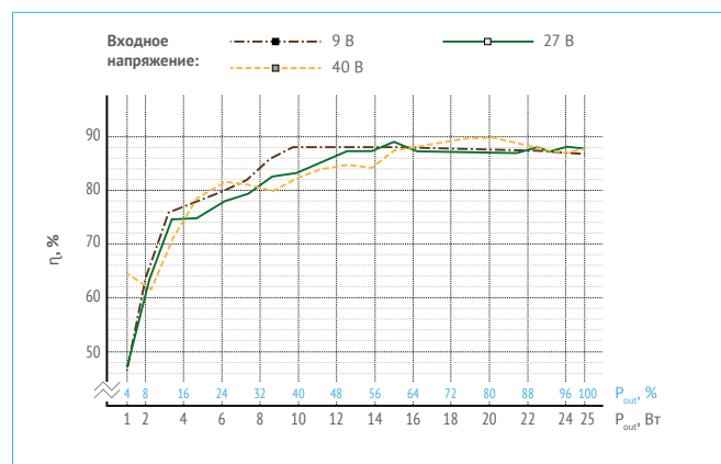
Рис. 14. МДМ25-1B12PC.
