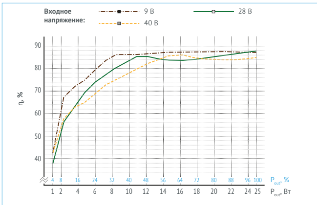
Рис. 17. МДМ25-1Б48РС.
