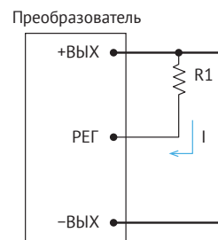
Рис. 10. Снижение Uвых.
