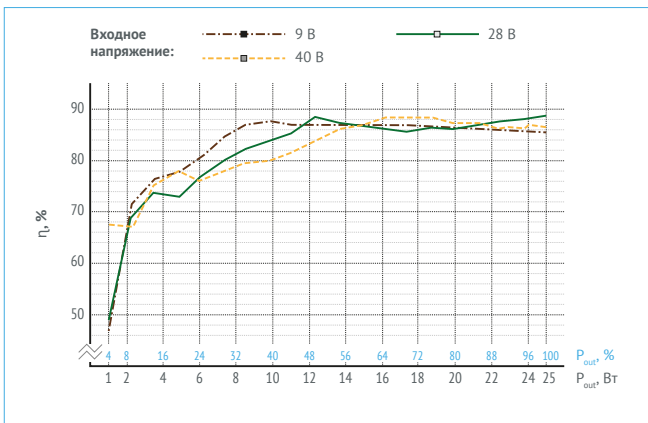
Рис. 13. МДМ25-1Б09РС.
