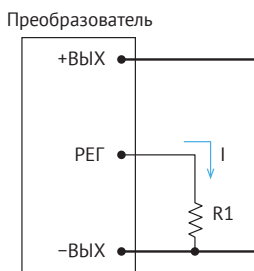
Рис. 9. Увеличение Uвых.
