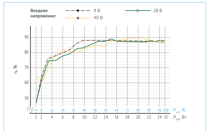
Рис. 14. МДМ25-1Б12РС.
