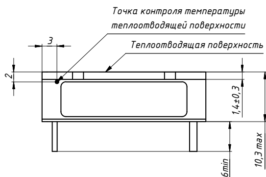
Рис. 21. Исполнение МДМ50-С.
