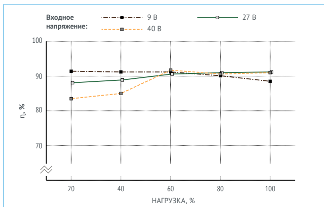
Рис. 10. МДМ50-1Б05РДС.
