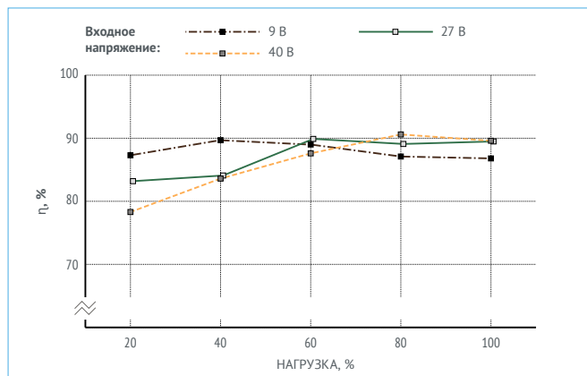
Рис. 11. МДМ50-1Б09РДС.
