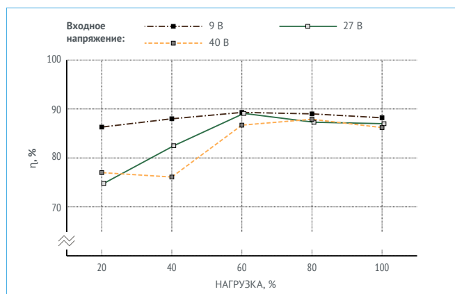
Рис. 13. МДМ50-1Б15РДС.
