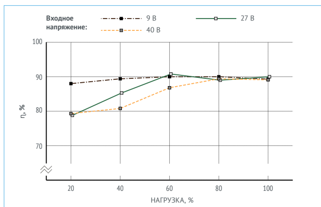
Рис. 12. МДМ50-1Б12РДС.
