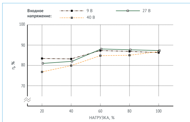
Рис. 14. МДМ50-1Б24РДС.
