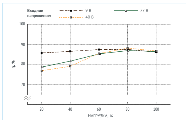
Рис. 15. МДМ50-1Б27РДС.
