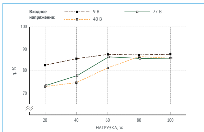
Рис. 16. МДМ50-1Б48РДС.
