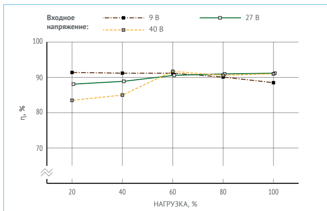
Рис. 10. МДМ50-1B05PDS.
