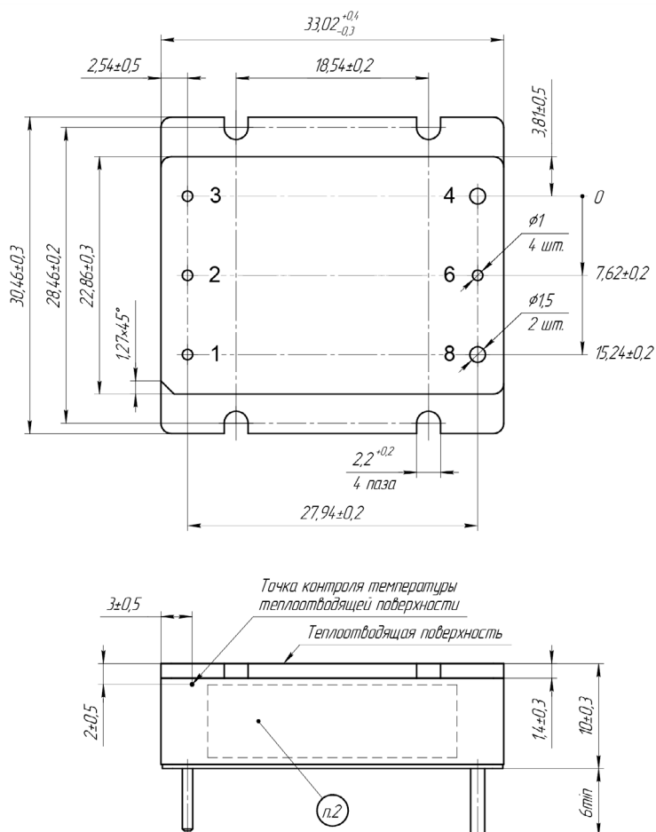
Рис. 21. Исполнение МДМ50-С.
