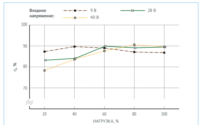
Рис. 11. МДМ50-1Б09РДС.
