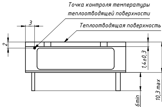
Рис. 21. Исполнение МДМ50-С.
