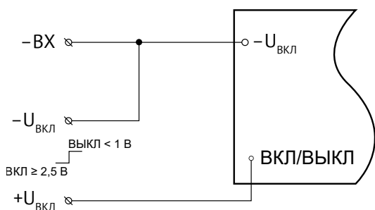
Рис. 7. Управление логическим напряжением.
