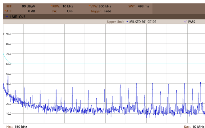
Рис. 22. Спектрограмма 0,15–10 MHz.
