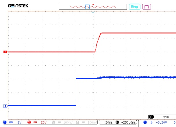
Рис. 18. Установление U_{\text{вых.ном}} с момента подачи U_{\text{вх.ном}} .
