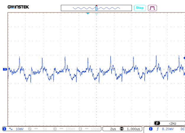
Рис. 19. Пульсации U_{ВЫХ.НОМ} .
