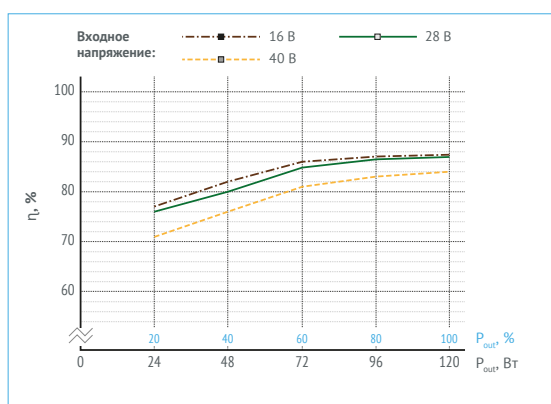
Рис. 16. МДМ120-1В48РДС.
