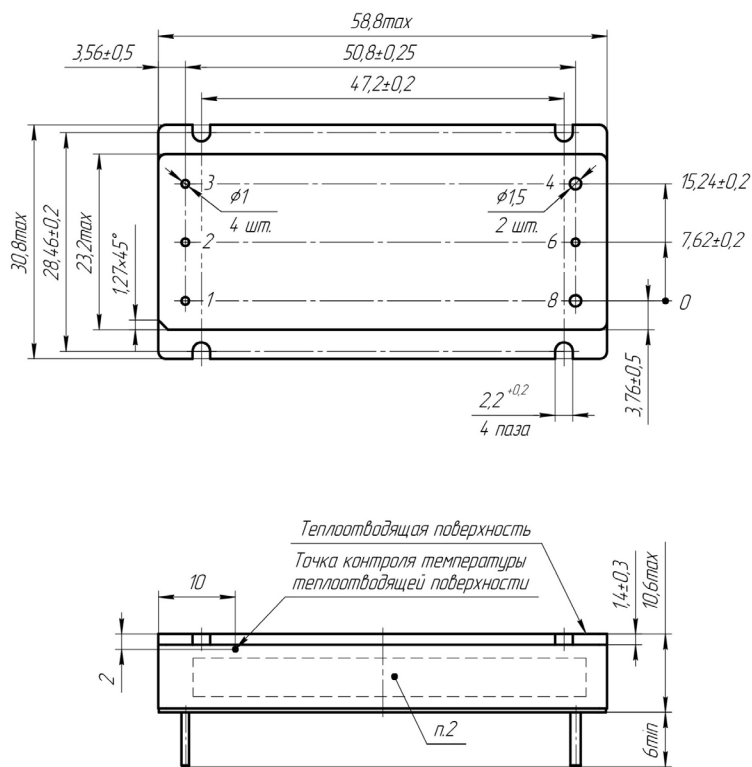
Рис. 23. Исполнение МДМ120-С.
