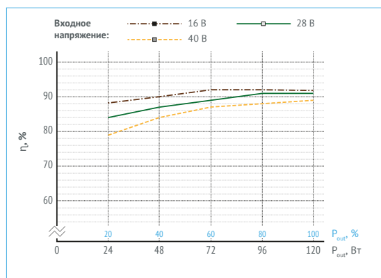
Рис. 13. МДМ120-1В15РДС.
