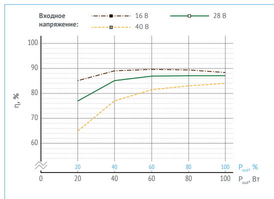
Рис. 11. МДМ120-1В05РДС.
