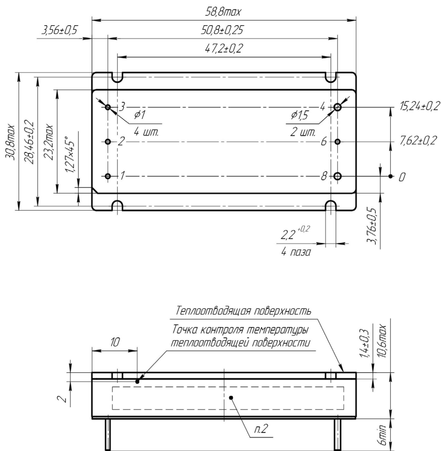
Рис. 23. Исполнение МДМ120-С.
